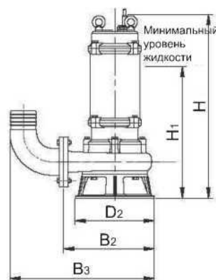
Погружная мобильная установка с коленом с резьбой
