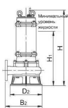
Погружная мобильная установка
