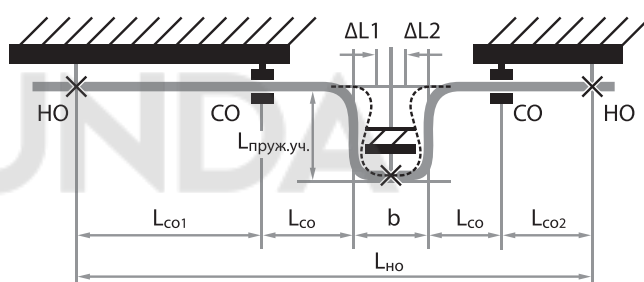
П-образный компенсатор
