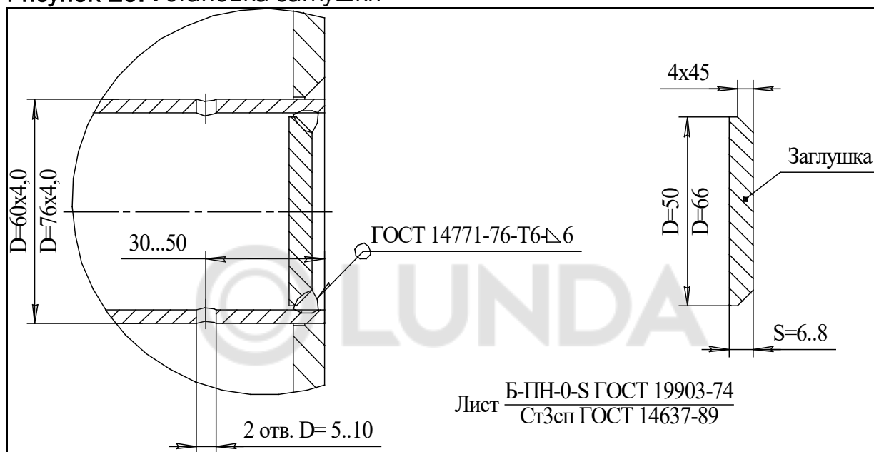
Рисунок 10. Установка заглушки
