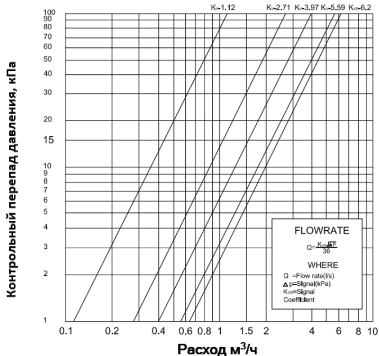
Клапан 1206 DN20
