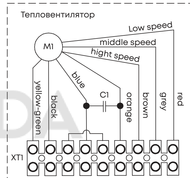
Внутренняя схема клеммной коробки тепловентилятора.
