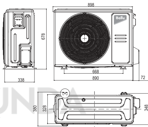
Размеры внешних блоков BM3OI-FM/out-21HN8_V1/EU:
