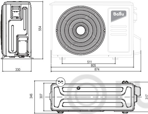
Размеры внешних блоков BM2OI-FM/out-14HN8_V1/EU, BM2OI-FM/out-18HN8_V1/EU:
