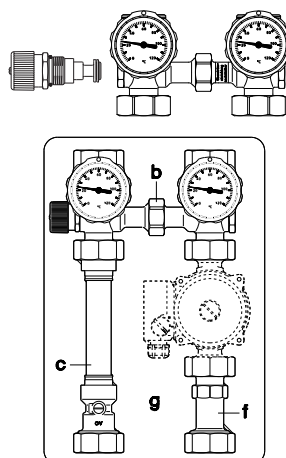
Перепускной клапан в „Regumat”
