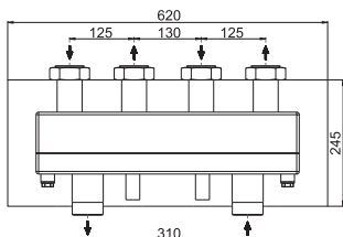
„HydroFixx” Ду32, на 2 группы
