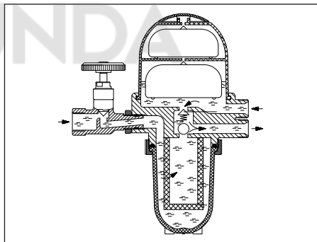
Схема работы „Tos-Duo”
