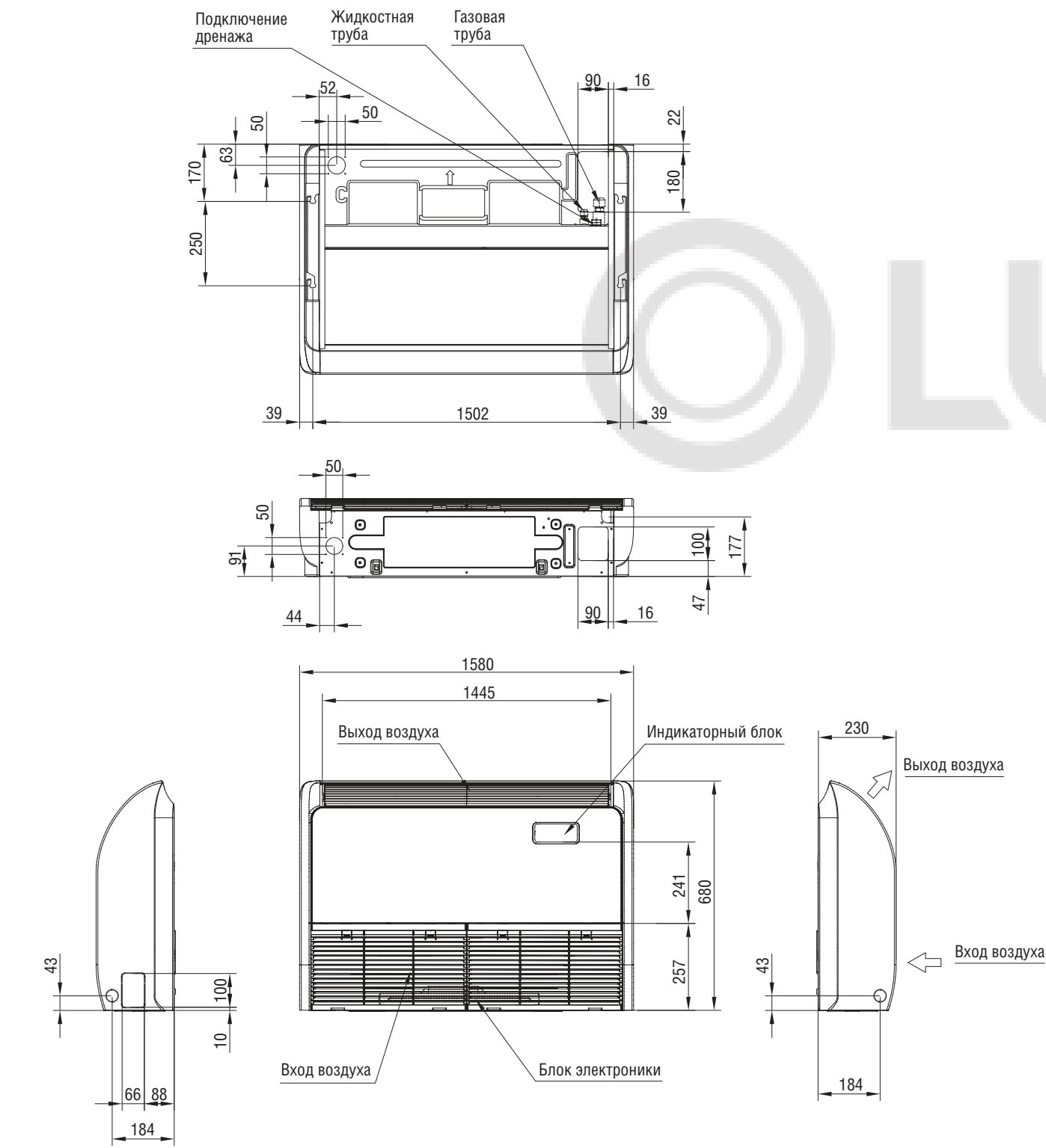
Блоки напольно-потолочного типа, модели 24/36/48/60
