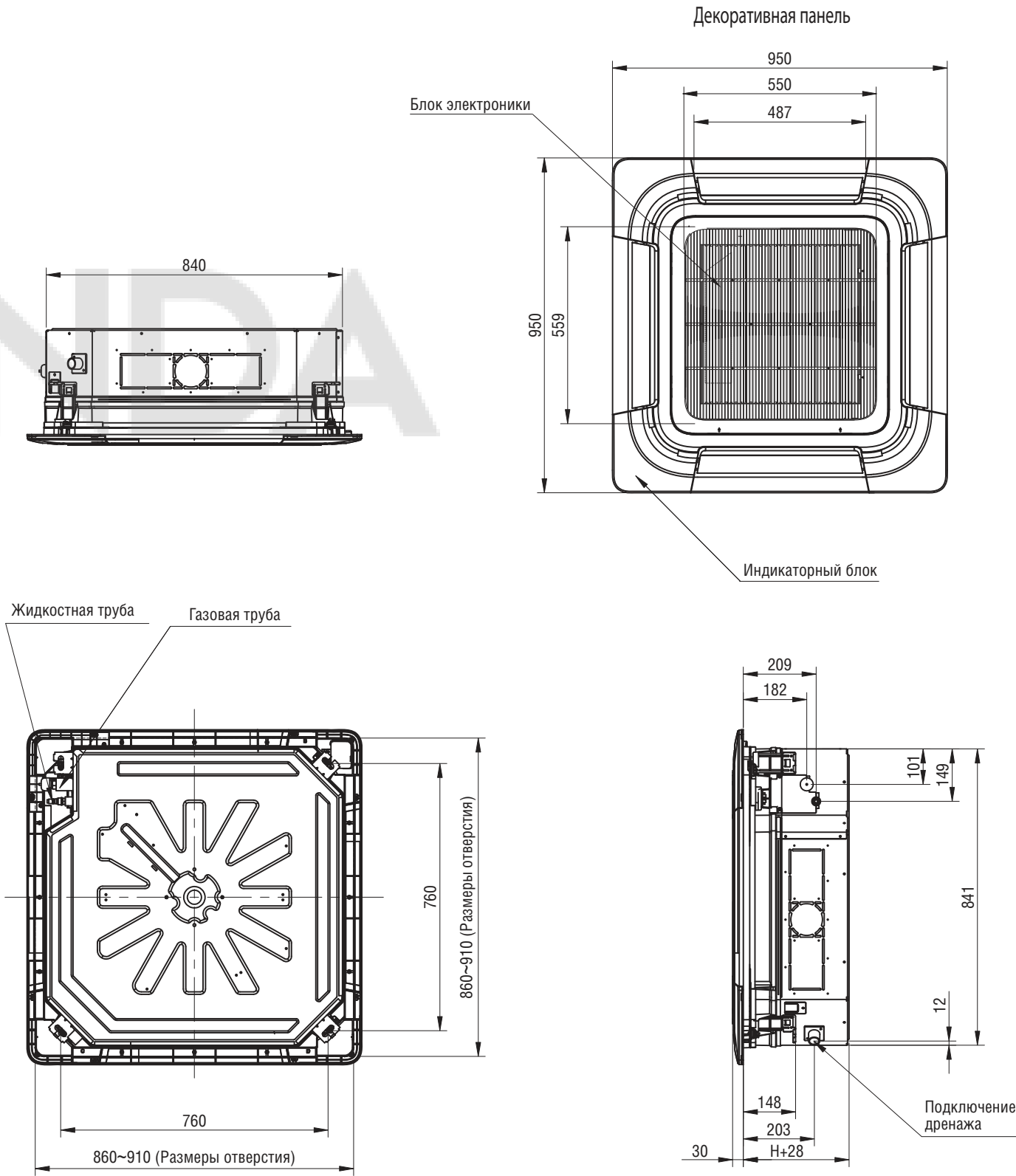
Блоки кассетного типа, модель 24/36/48/60
