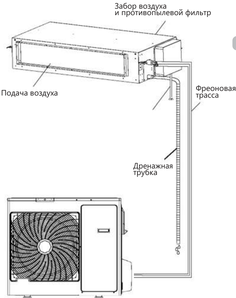
Наружный блок (типоразмер 9/12/18/24/36/60)
