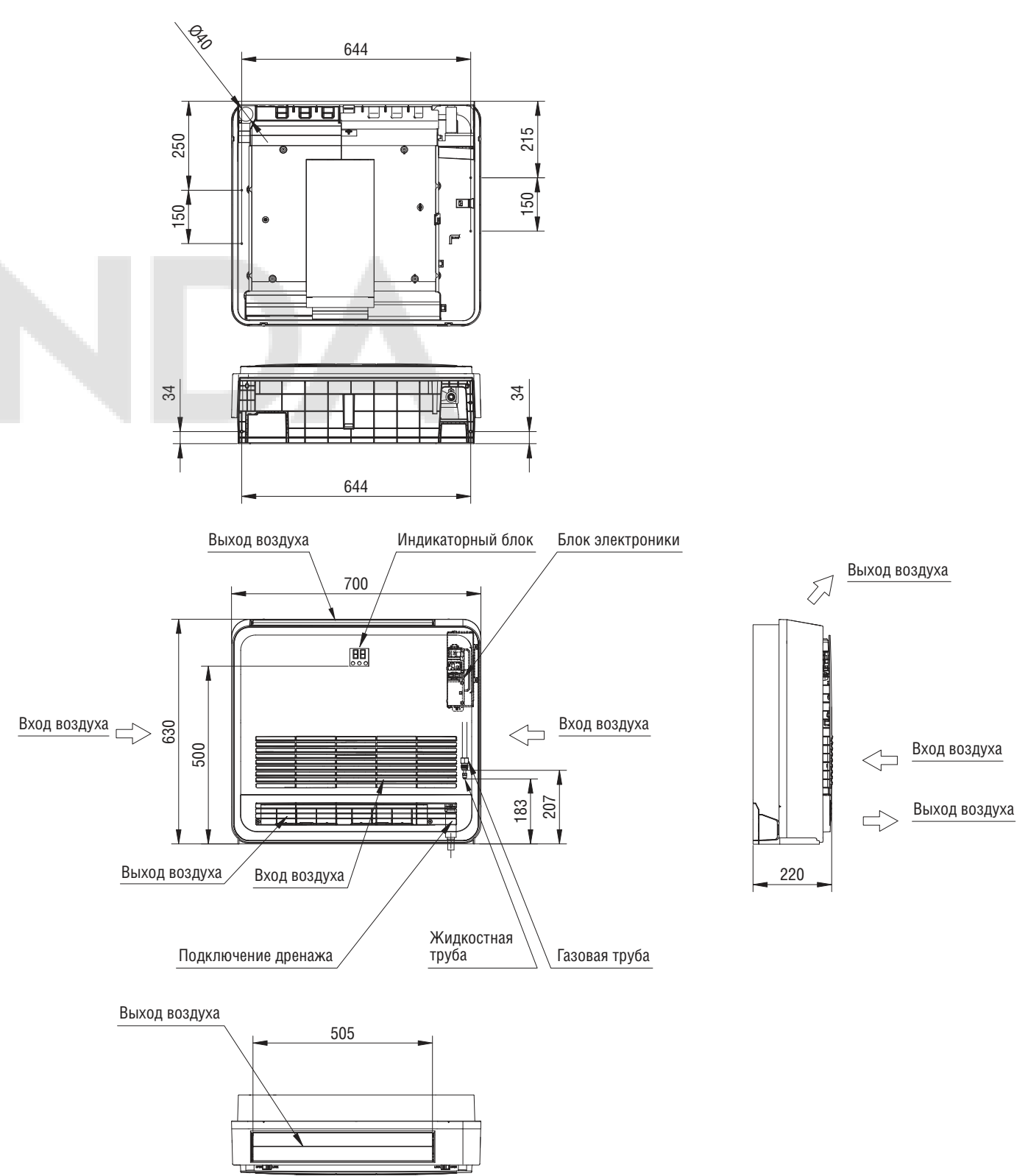
Блоки консольного типа, модели 9/12
