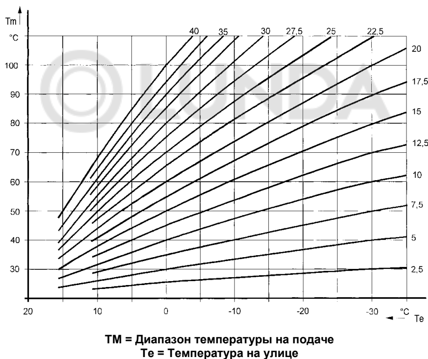
Рис. 31: Выбор рабочей кривой датчика уличной температуры при наличии климатического регулятора QAA 73
