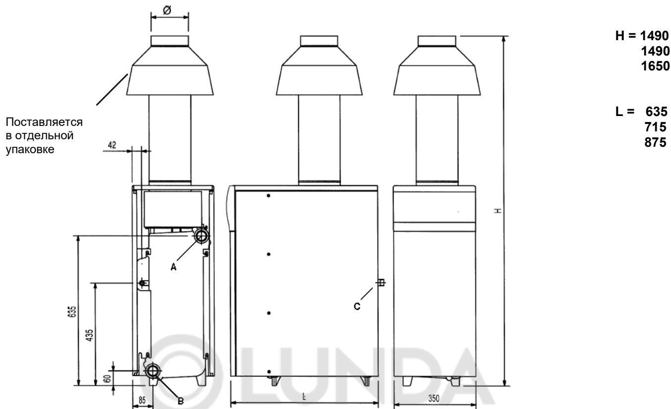
Рис. 4: Габаритные размеры для моделей 1.400 iN, 1.490iN, 1.620iN
