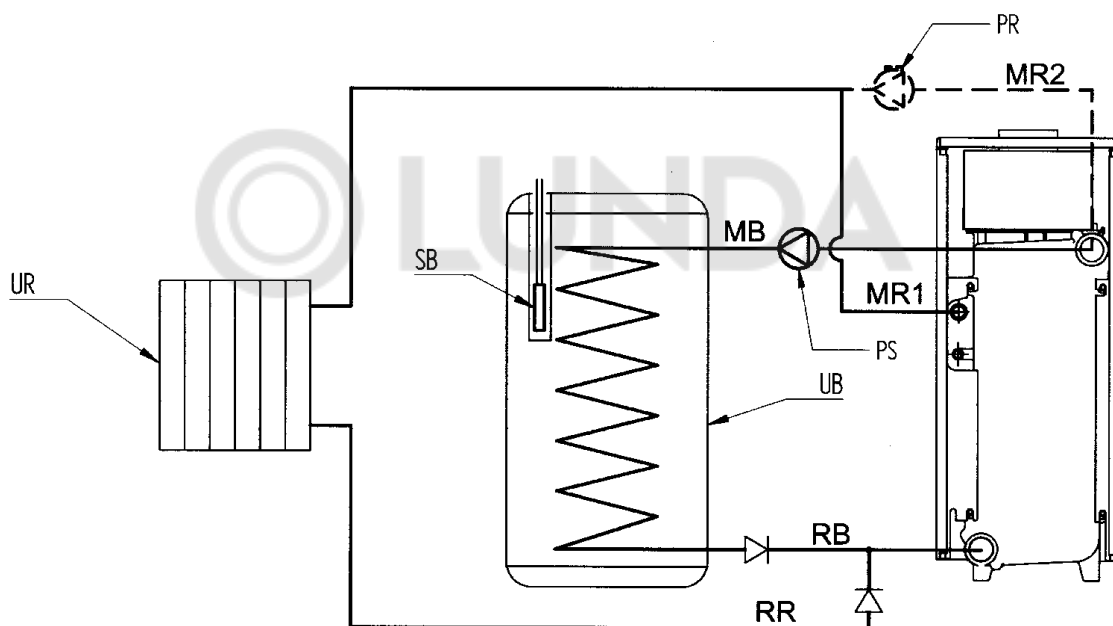
Рис. 24: Схема гидравлического присоединения бойлера
