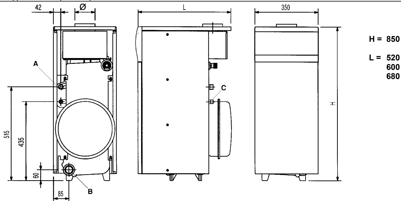
Рис. 5: Габаритные размеры для моделей 1.150 i, 1.230 i, 1.300 i
