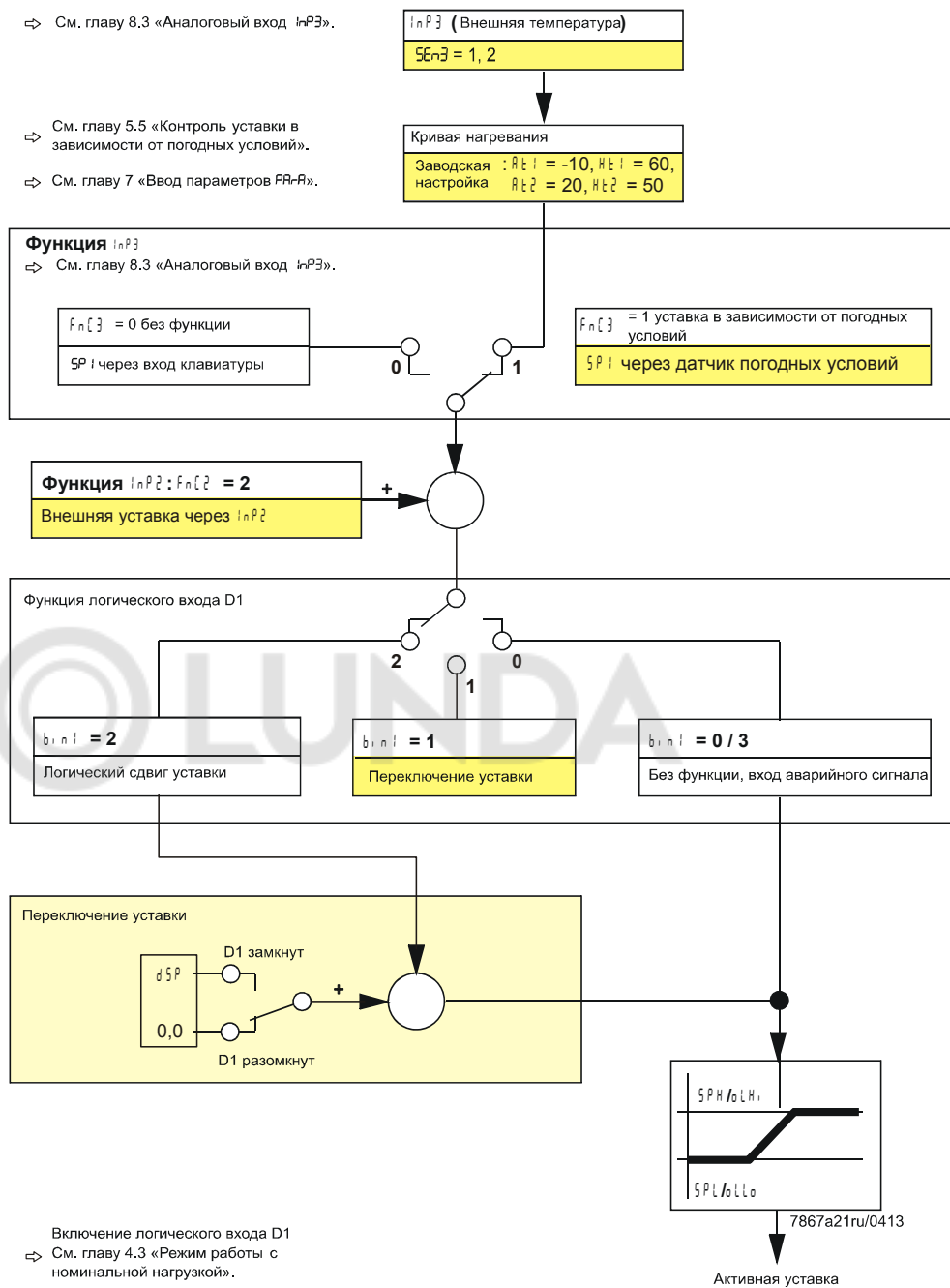
График 14: Сдвиг уставки аналоговый/логический
