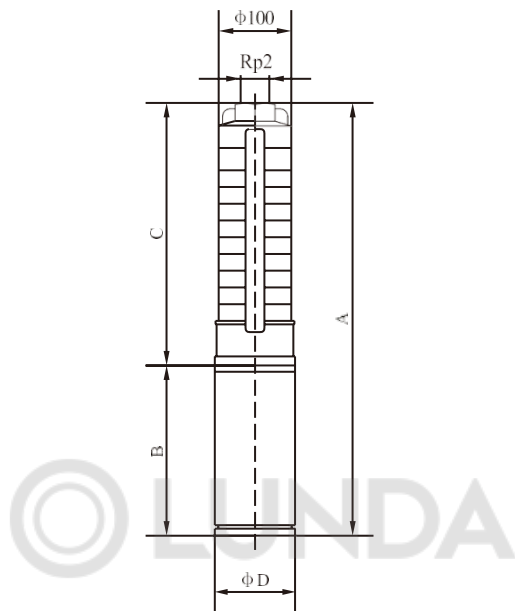
Рис. Б.4 Габаритно-присоединительные размеры насосных агрегатов SJ 8
