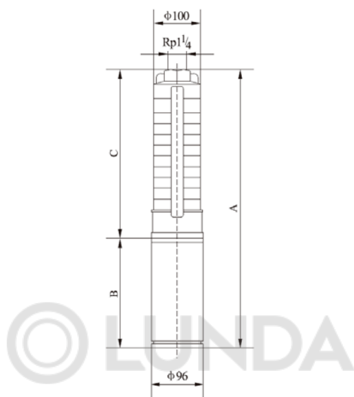
Рис. Б.2 Габаритно-присоединительные размеры насосных агрегатов SJ 3
