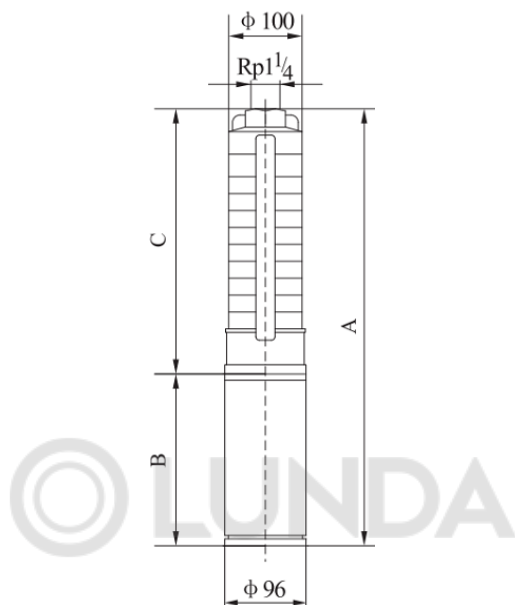
Рис. Б.1 Габаритно-присоединительные размеры насосных агрегатов SJ 1
