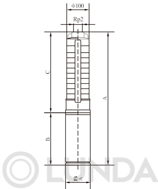
Рис. Б.5 Габаритно-присоединительные размеры насосных агрегатов SJ 12
