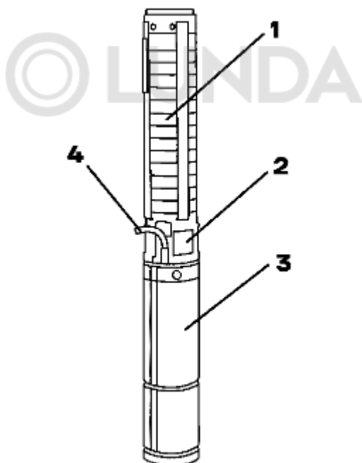
Рис. 1 Структура насосного агрегата SJ.
