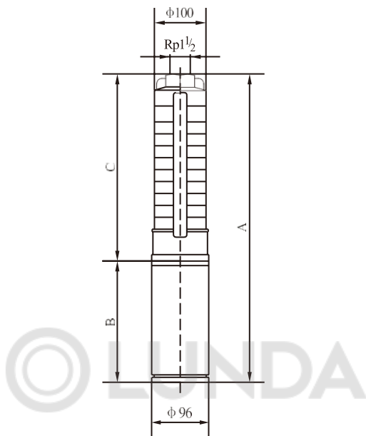
Рис. Б.3 Габаритно-присоединительные размеры насосных агрегатов SJ 5
