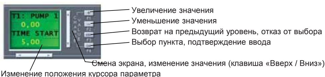
Рис. 1. Работа с кнопками управления логического модуля
