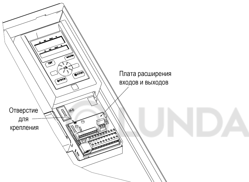
Рисунок 4.1 – Монтаж платы расширения входов и выходов
