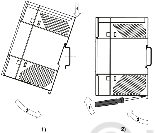
Рисунок 4 – Монтаж (1) и демонтаж (2) прибора
