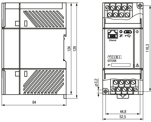
Рисунок 3 – Габаритные и установочные размеры прибора
