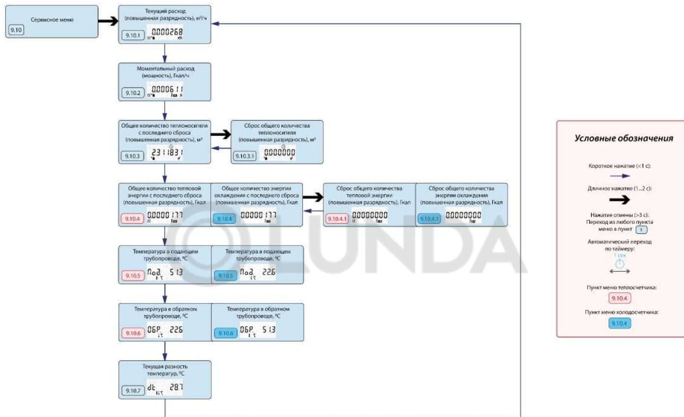
Рисунок 16 — Структура меню поверки теплосчетчика или холодосчетчика
