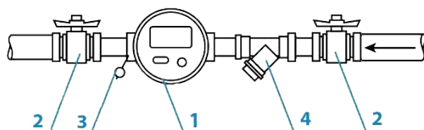
Рисунок 7 — Схема монтажа
