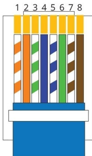
Рисунок 11 — Новая распиновка
