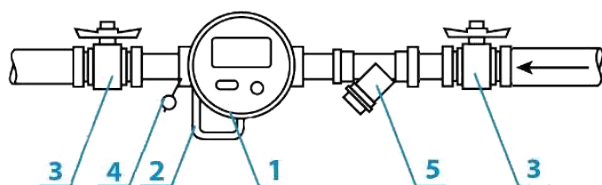
Рисунок 8 — Схема монтажа
