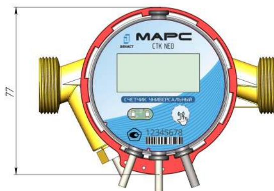
Рисунок 4 — Габаритные размеры СТК MAPC NEO (иные модификации)
