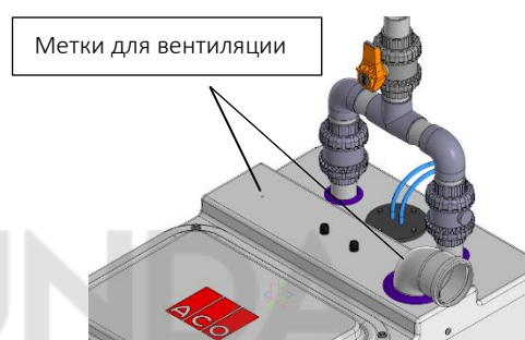
Рисунок 14 – Подключение вентиляции
