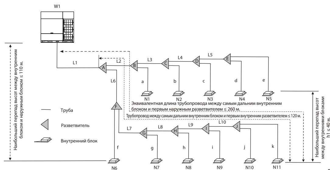
Схема трубопровода индивидуальных блоков серии V8i
