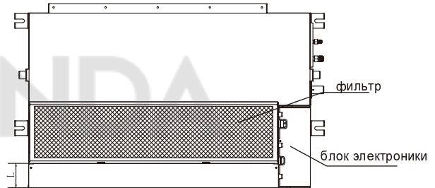
Размеры во входу воздуха (вход воздуха снизу):
