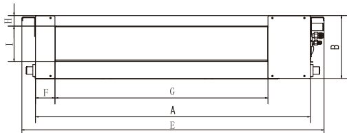
Размеры во входу воздуха (вход воздуха сзади):
