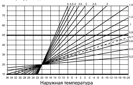
Температура подачи
