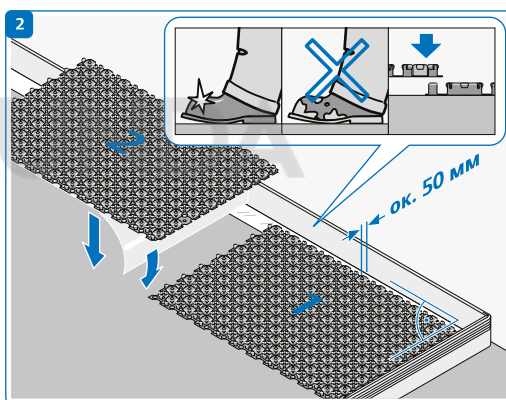
Укладка панелей
