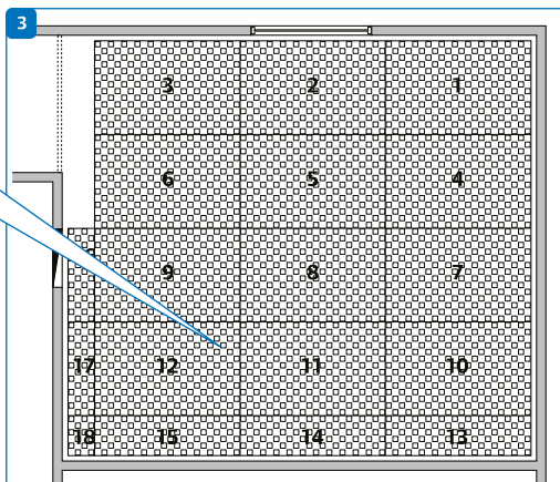
Укладка панелей
