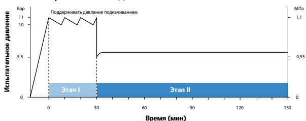
График проведения гидравлических испытаний системы Uropor MLC водой
