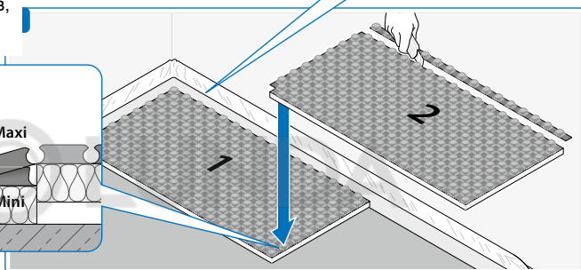
Укладка панелей
