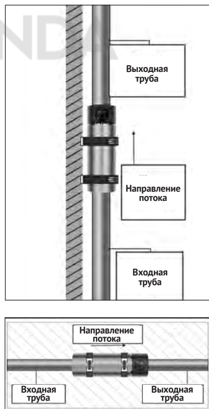
Рисунок 3 – Вертикальная или горизонтальная установка
