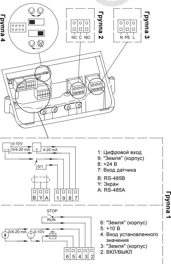
Рис. 5 Клеммы насосов TPED
