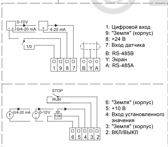
Рис. 8 Клеммы насосов TPE, NKE, NKGE и NBE, NBGE
