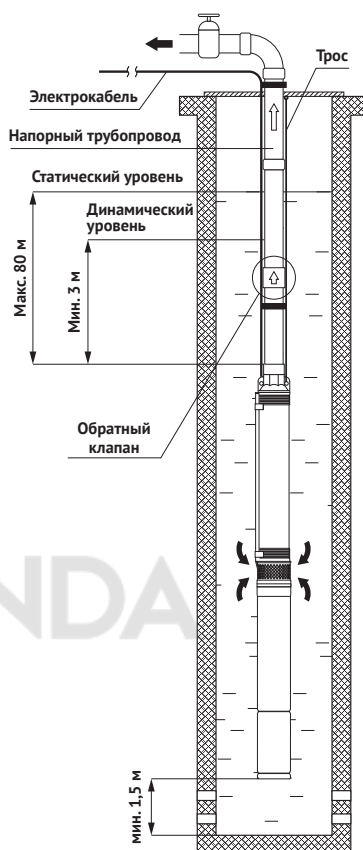
Рисунок 4 - Установка насоса
