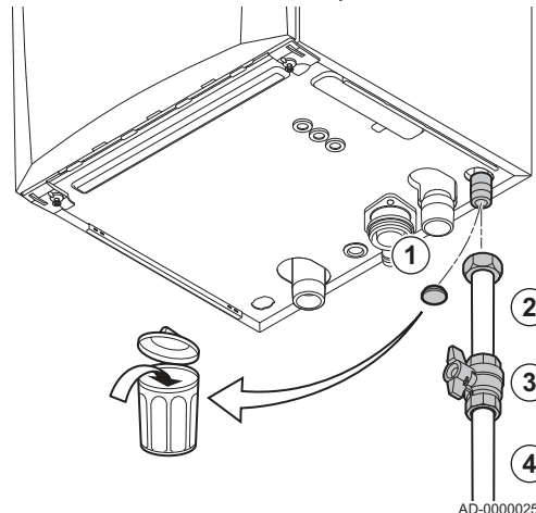
Рис.18 Подключение газопровода
