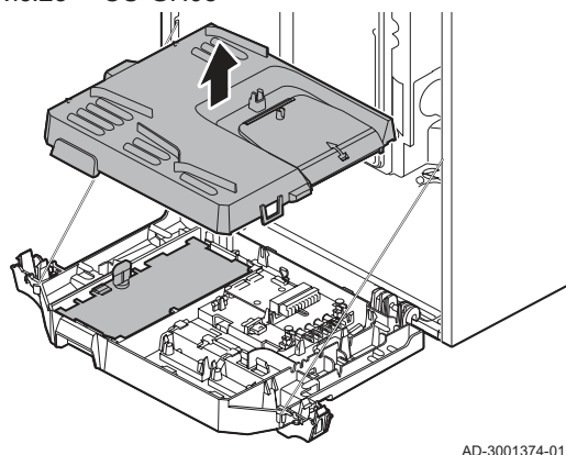
Рис.23 CU-GH08
