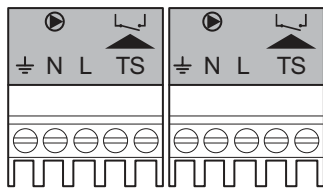
Рис.39 Разъём насоса с защитным термостатом
