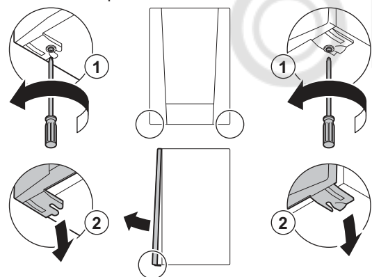
Рис.68 Открытие котла
