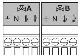
Рис.38 Разъёмы смесительного клапана
