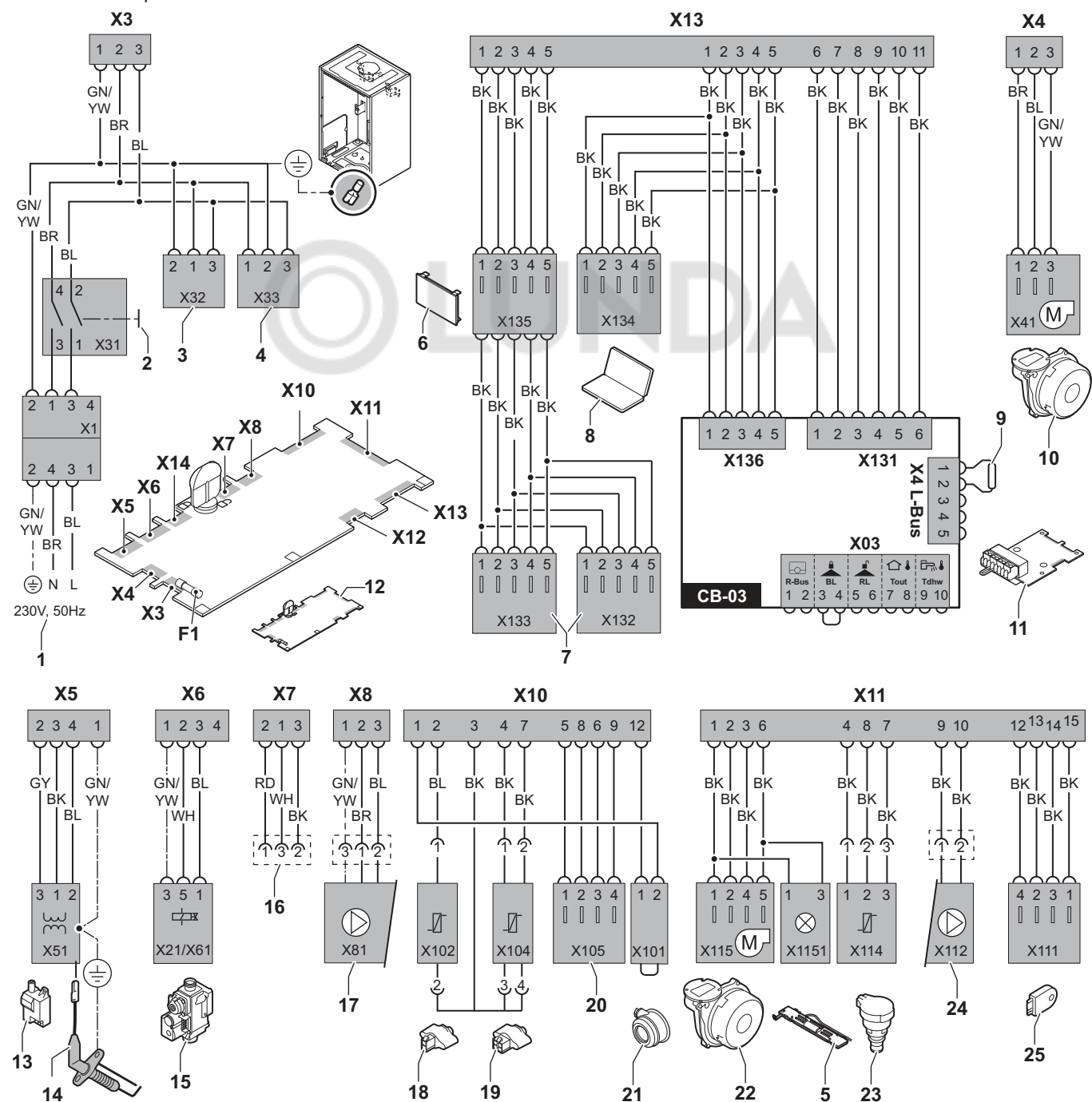
Рис.82 Электрическая схема
