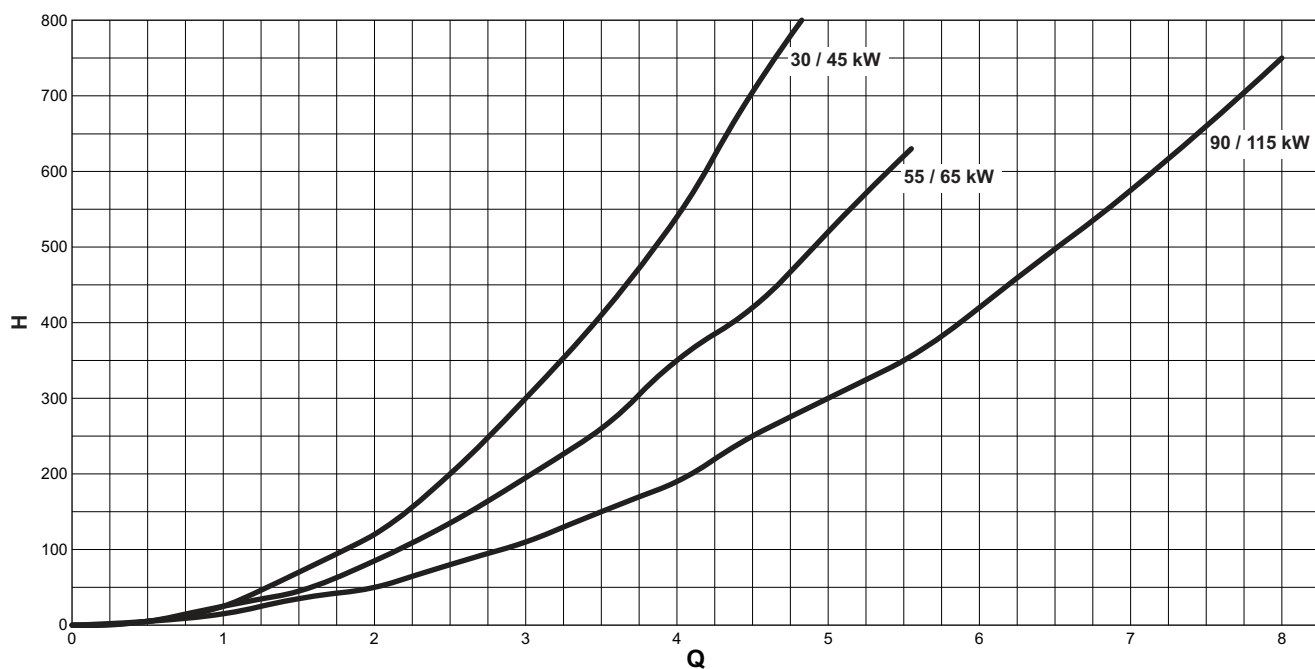
Рис.84 Гидравлическое сопротивление
