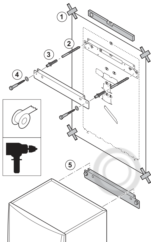
Рис.15 Установка котла
