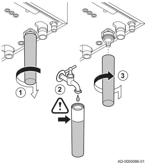
Рис.50 Заполнение сифона
