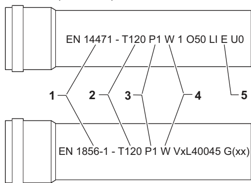
Рис.5 Простая строка
