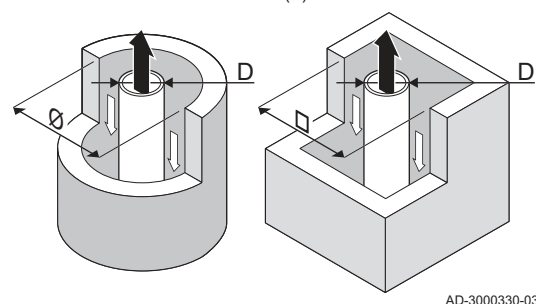
Рис.4 Минимальные размеры шахты или канала C 93(X)
