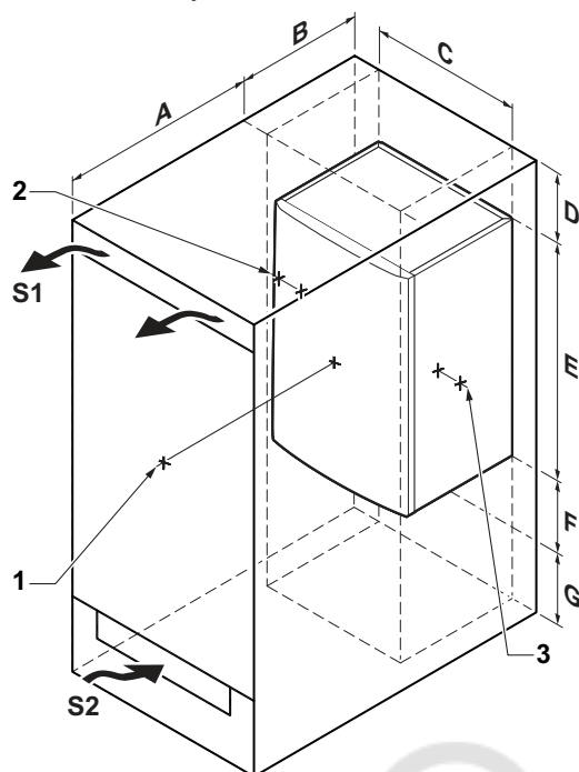
Рис.3 Зона установки
