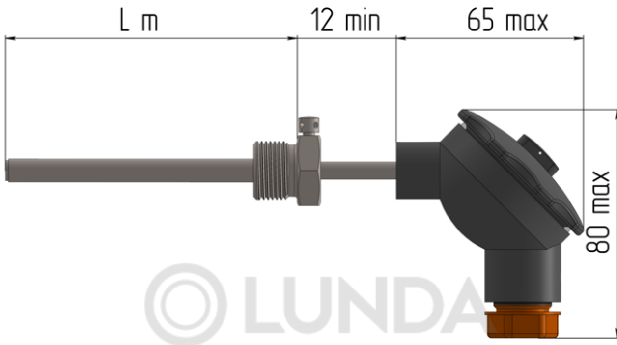
Рисунок 1а – Датчик температуры ТДТА.
