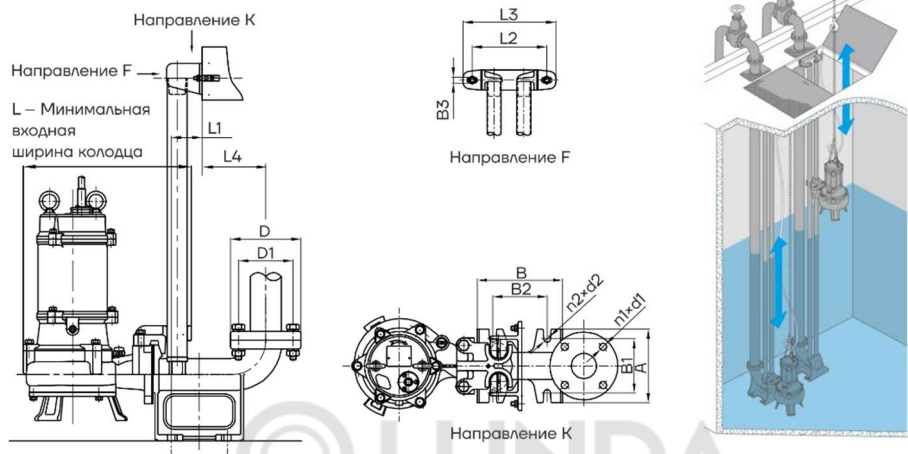
Рис. 17а – Стационарная установка носов серии WQ при помощи автоматической трубной муфты
