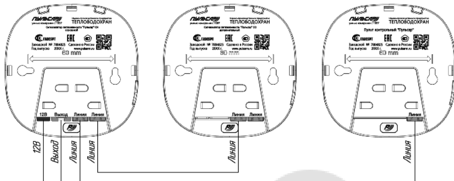
Сигнализатор загазованности "Пульсар" СН основной
