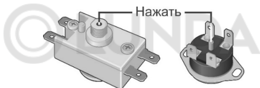
Рисунок 2. Схема расположения кнопки термовыключателя
