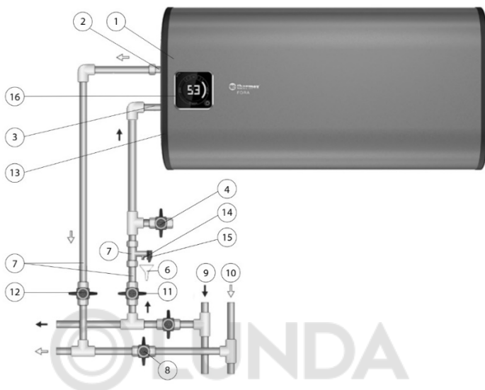
Рисунок 2. Схема подключения ЭВН к водопроводу в горизонтальном положении
