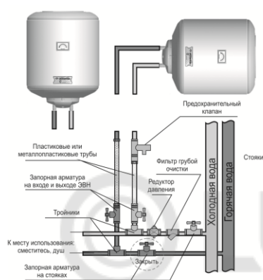
Рис. 5. Подключение ЭВН в вертикальном / горизонтальном положении
