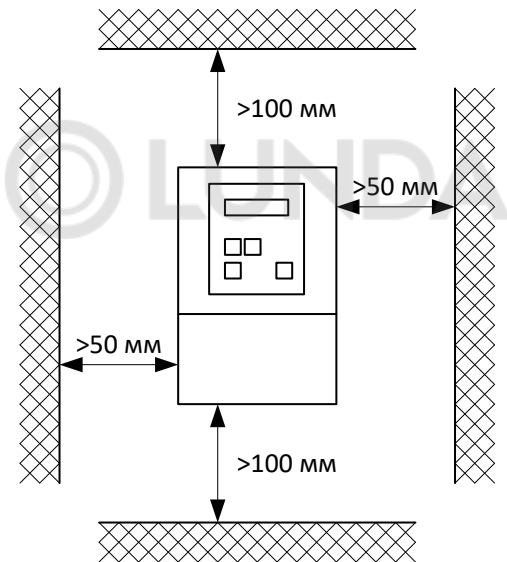
Рисунок 3 – Установка ПЧ
