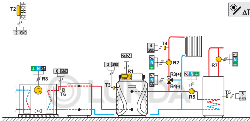
Схема 422с (W20) - Тепловой насос, ЖТ котел, бак-теплоаккумулятор, смесительный контур р, бойлер ГВС
