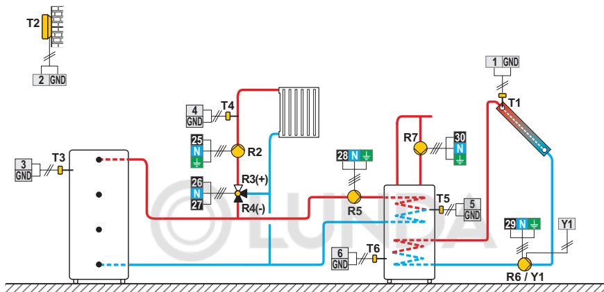
Схема 404b (W10, W20) - Бак-теплоаккумулятор, смесительный контур, бойлер ГВС, солнечный коллектор
