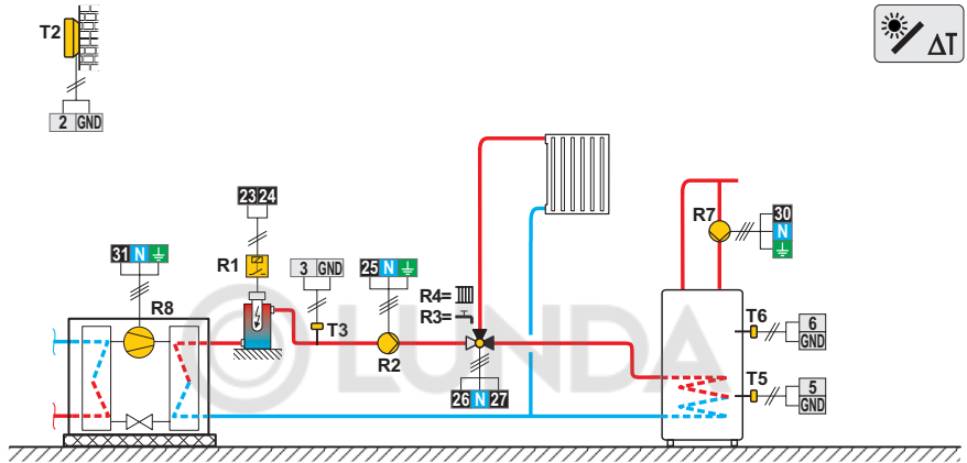
Схема 420 (W20) - Тепловой насос, дополнительный электрический нагреватель, прямой контур, бойлер ГВС
