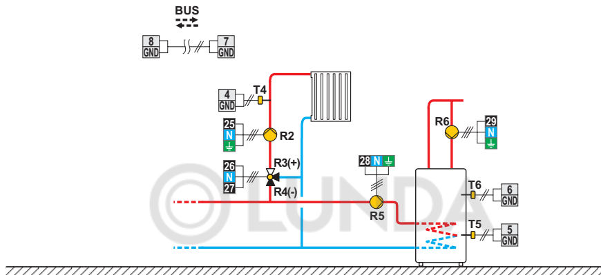
Схема 402 (W10B, W10, W20) - ЖТ котел, прямой контур, бойлер ГВС
