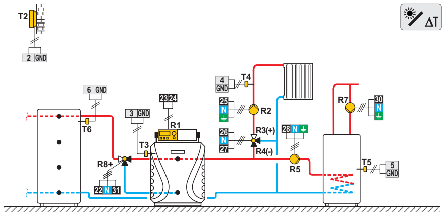
Схема 421 (W20) - ЖТ котел, бак-теплоаккумулятор, смешивательный контур, бойлер ГВС
