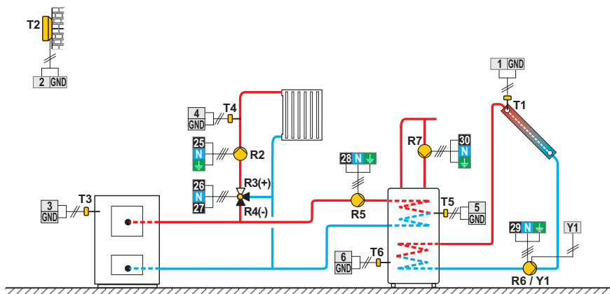
Схема 404c (W10, W20) - ТТ котел, смесительный контур, бойлер ГВС, солнечный коллектор
