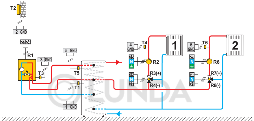
Схема 423с (W20) - Газовый котел, бак-теплоаккумулятор с встроенным бойлером ГВС, 2 смесительных контура
