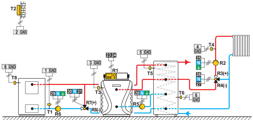
Схема 415с (W20) - ЖТ котел, ТТ котел, бак-теплоаккумулятор с встроенным бойлером ГВС, смесительный контур
