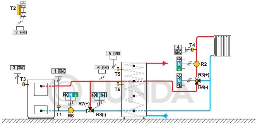
Схема 415б (W20) - ТТ котел, бак-теплоаккумулятор, смесительный контур, бойлер ГВС
