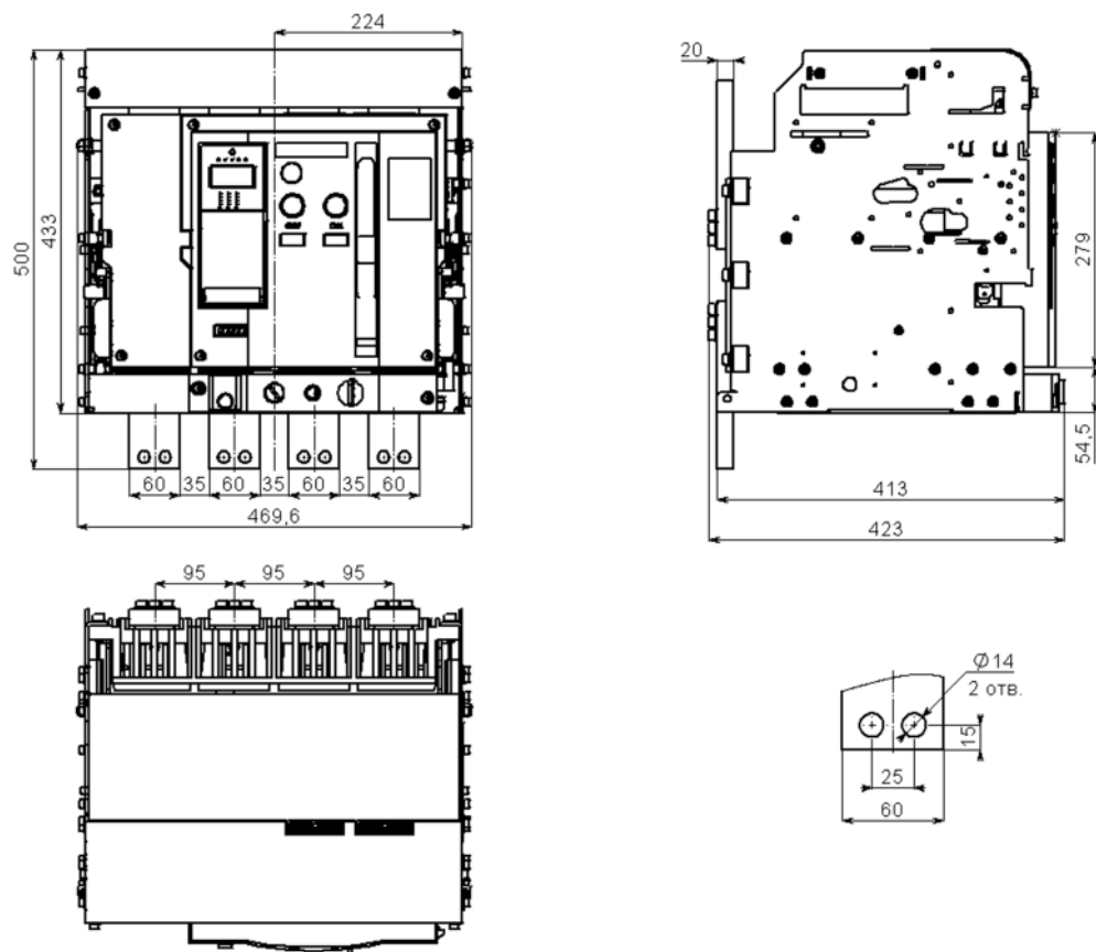
Рисунок А.18 – Автоматический выключатель YON AD-S2 выдвижного исполнения на номинальные токи 630–1600 А переднего присоединения 4 полюса
