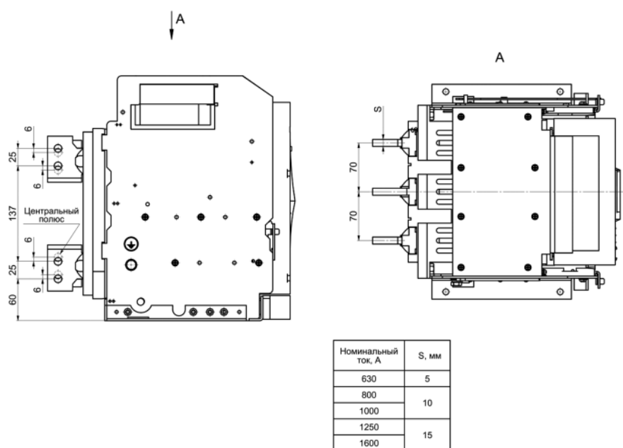
Рисунок А.29 – Автоматический выключатель YON AD1600-S1 выдвижного исполнения на номинальный ток 1600 А с расширителями полюсов
