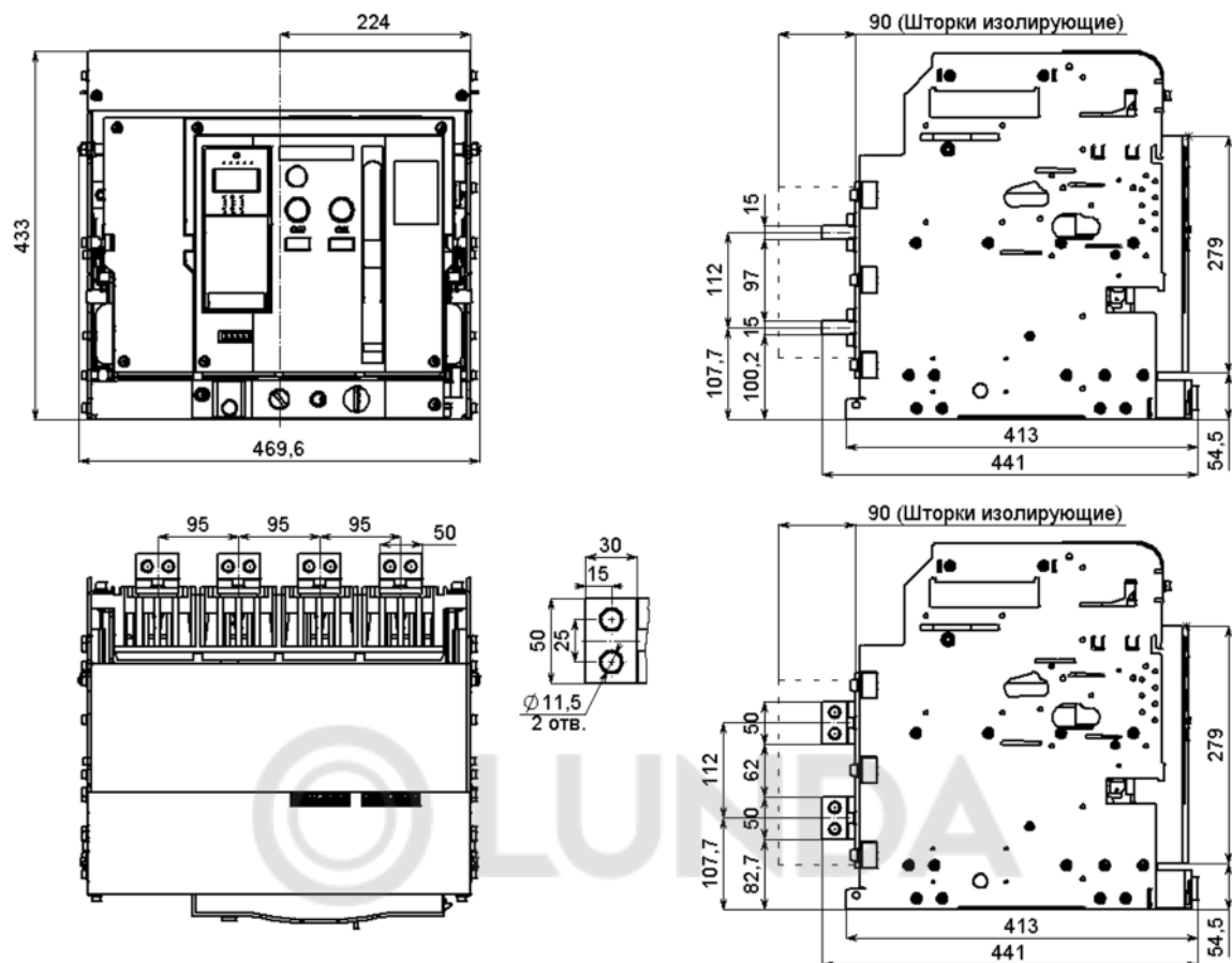
Рисунок А.17 – Автоматический выключатель YON AD-S2 выдвижного исполнения на номинальные токи 630–1600 А заднего присоединения 4 полюса
