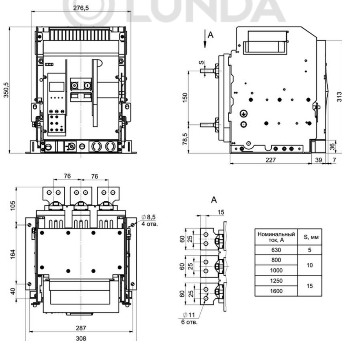
Рисунок А.28 – Автоматический выключатель YON AD630–1600–S1 выдвижного исполнения на номинальные токи 630 – 1600 А с горизонтальным расположением выводов
