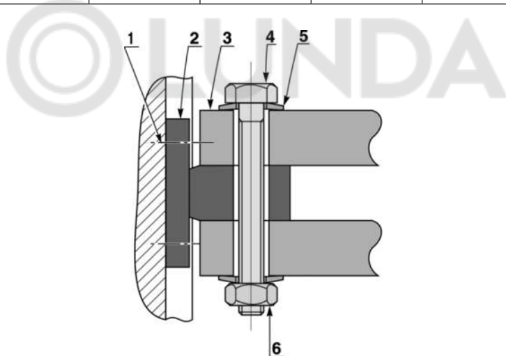
1 – винт крепления к аппарату; 2 – коннектор выключателя; 3 – шины; 4 – болт; 5 – пружины тарельчатые; 6 – гайка.
