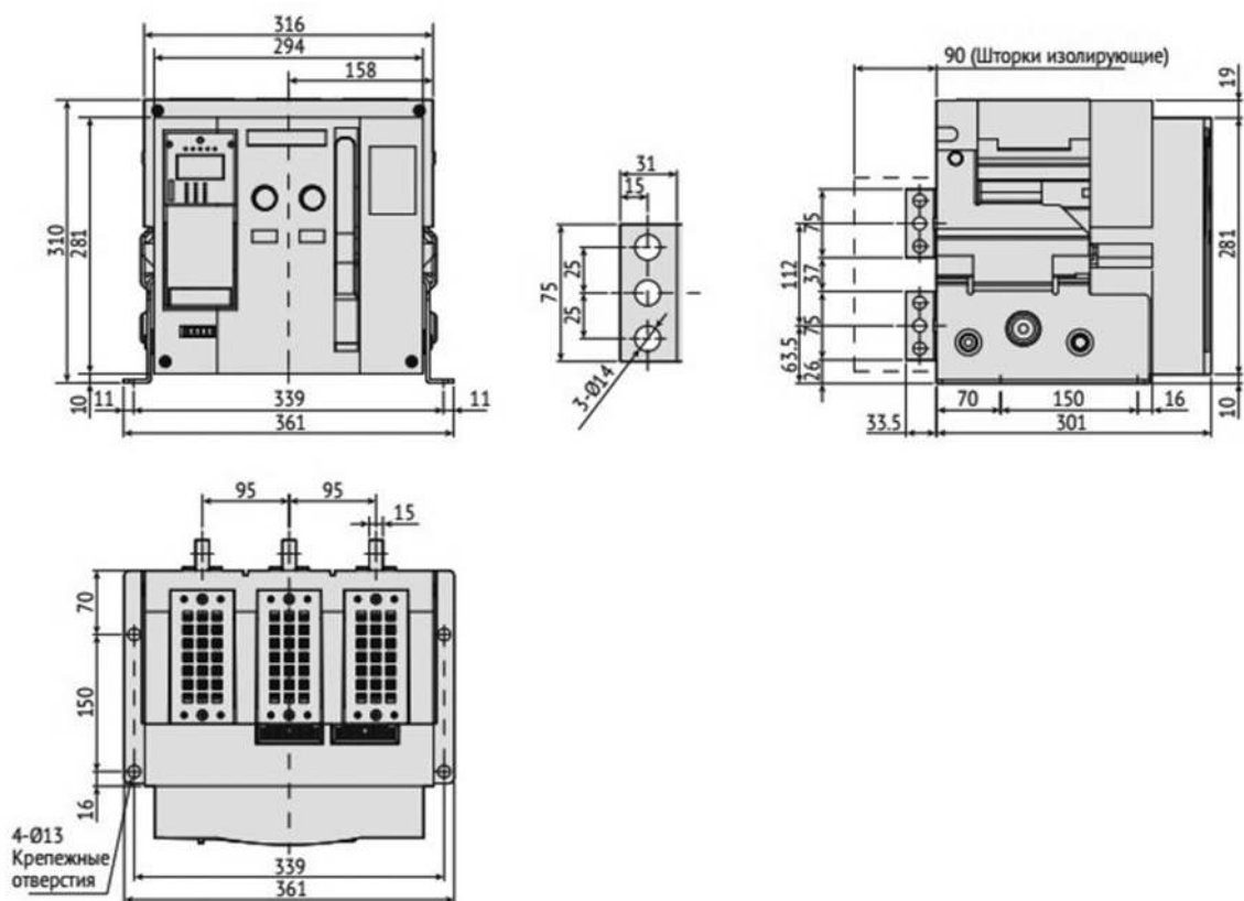
Рисунок А.2 – Автоматический выключатель YON AD-S2 стационарного исполнения на номинальный ток 2000 А заднего присоединения
