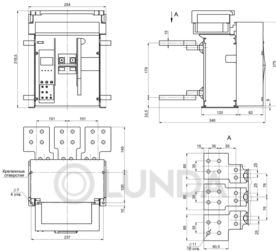
Рисунок A.25 – Автоматический выключатель YON AD1600-S1 стационарного исполнения на номинальный ток 1600 А с расширителями полюсов
