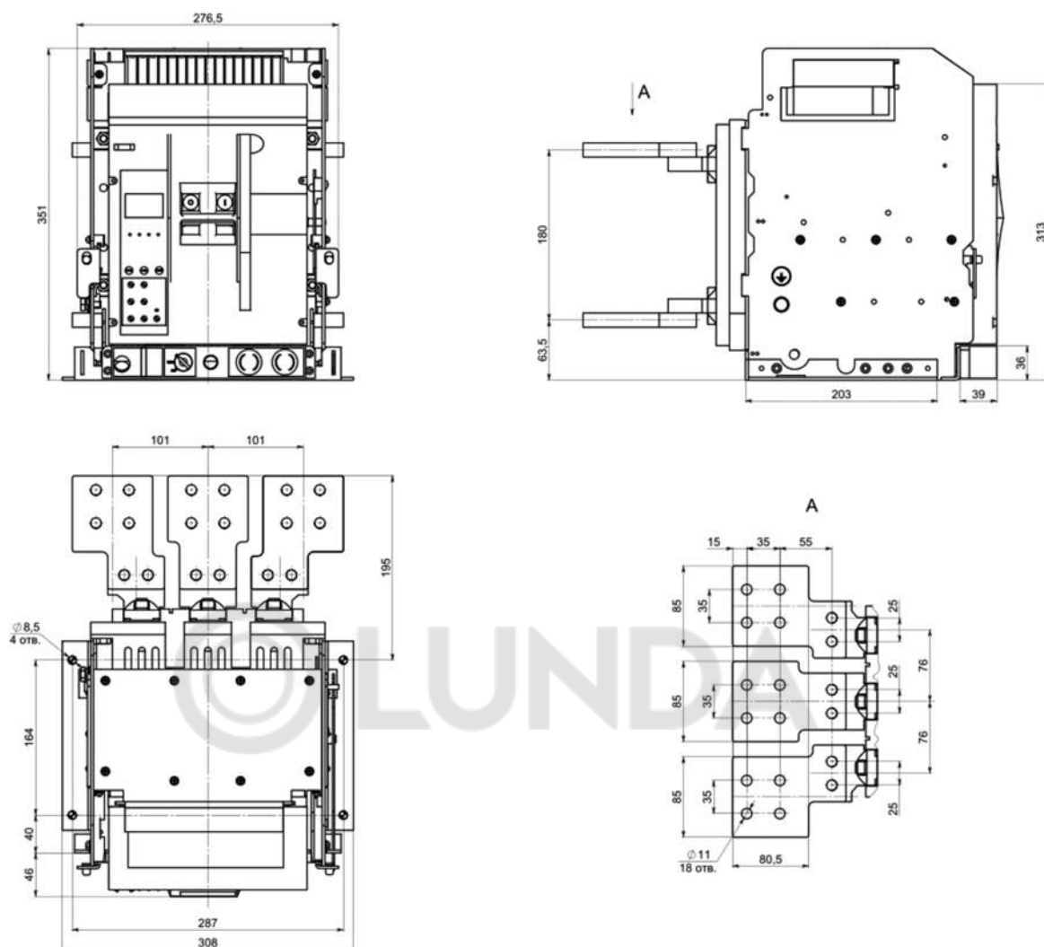
Рисунок А.29 – Автоматический выключатель YON AD1600-S1 выдвижного исполнения на номинальный ток 1600 А с расширителями полюсов
