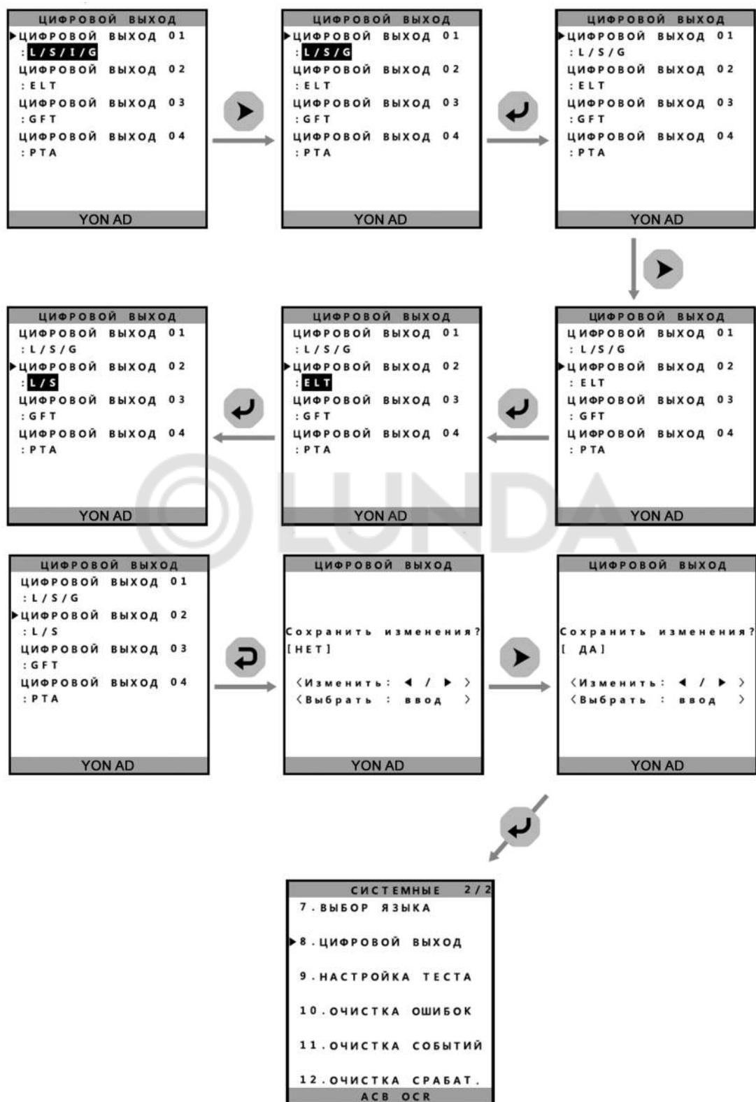
Рисунок 17 – «Системные-Цифровой выход»
