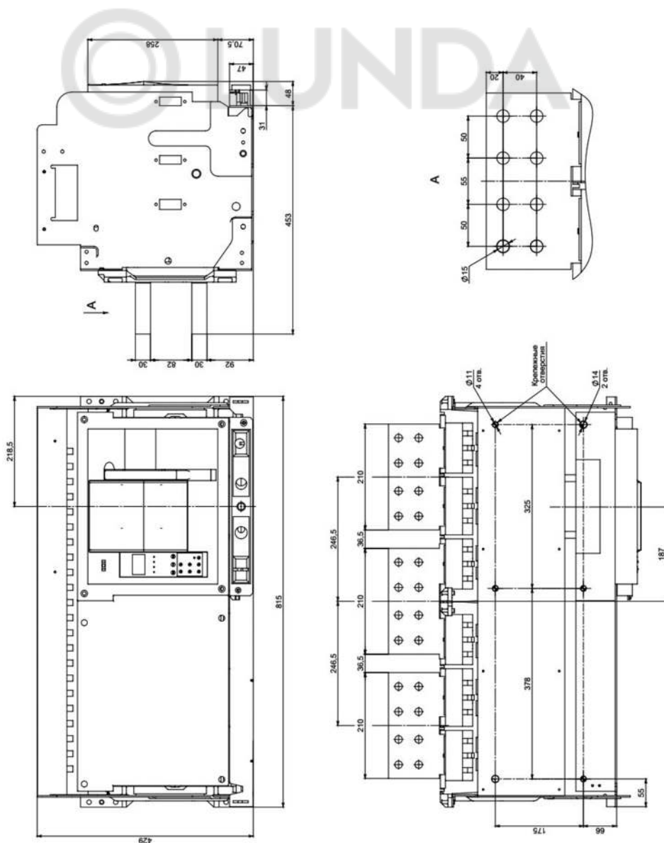
Рисунок А.31 – Автоматический выключатель YON AD5000-S5 выдвижного исполнения на номинальный ток 5000 А
