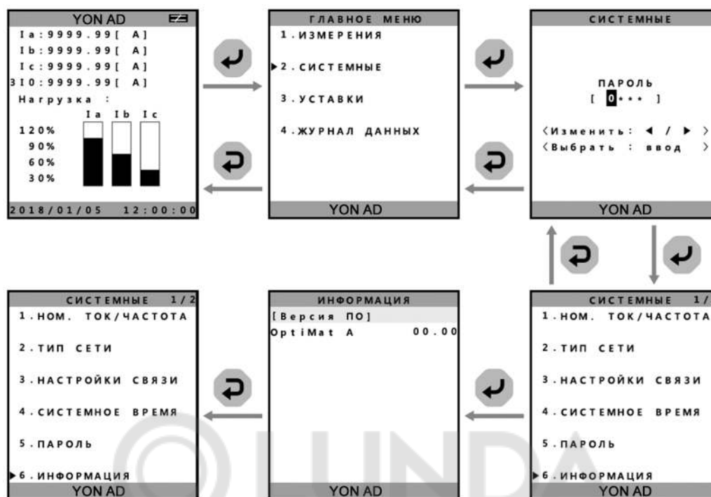
Рисунок 15 – «Системные-Информация»
