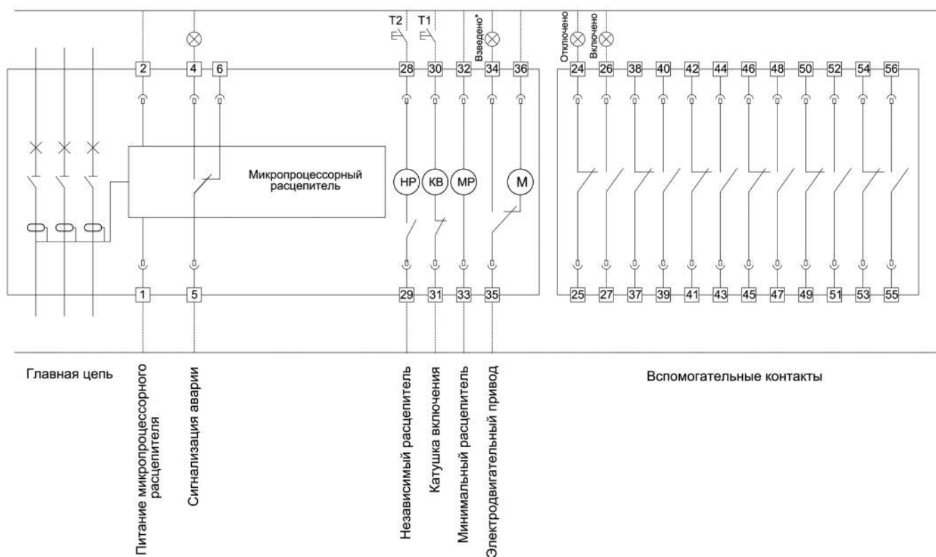
Рисунок В.5 - Схема электрическая принципиальная выключателя YON AD630-1600-S1 с электронным расцепителем MR5.0
