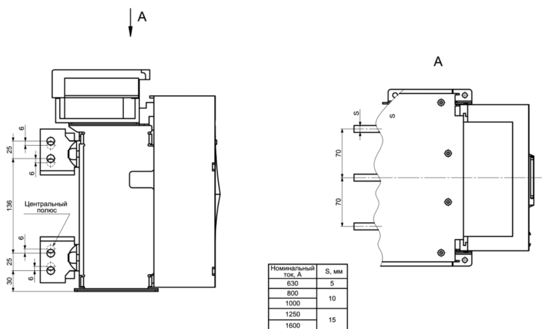
Рисунок A.26 – Автоматический выключатель YON AD630-1600-S1 стационарного исполнения на номинальные токи 630 – 1600 А с вертикальным расположением выводов
