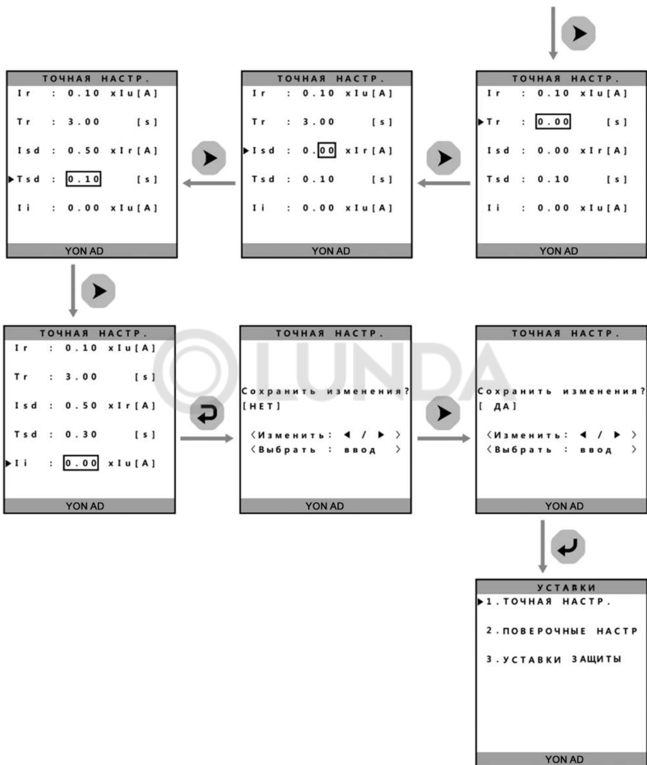
Рисунок 23 – «Точные настройки»
