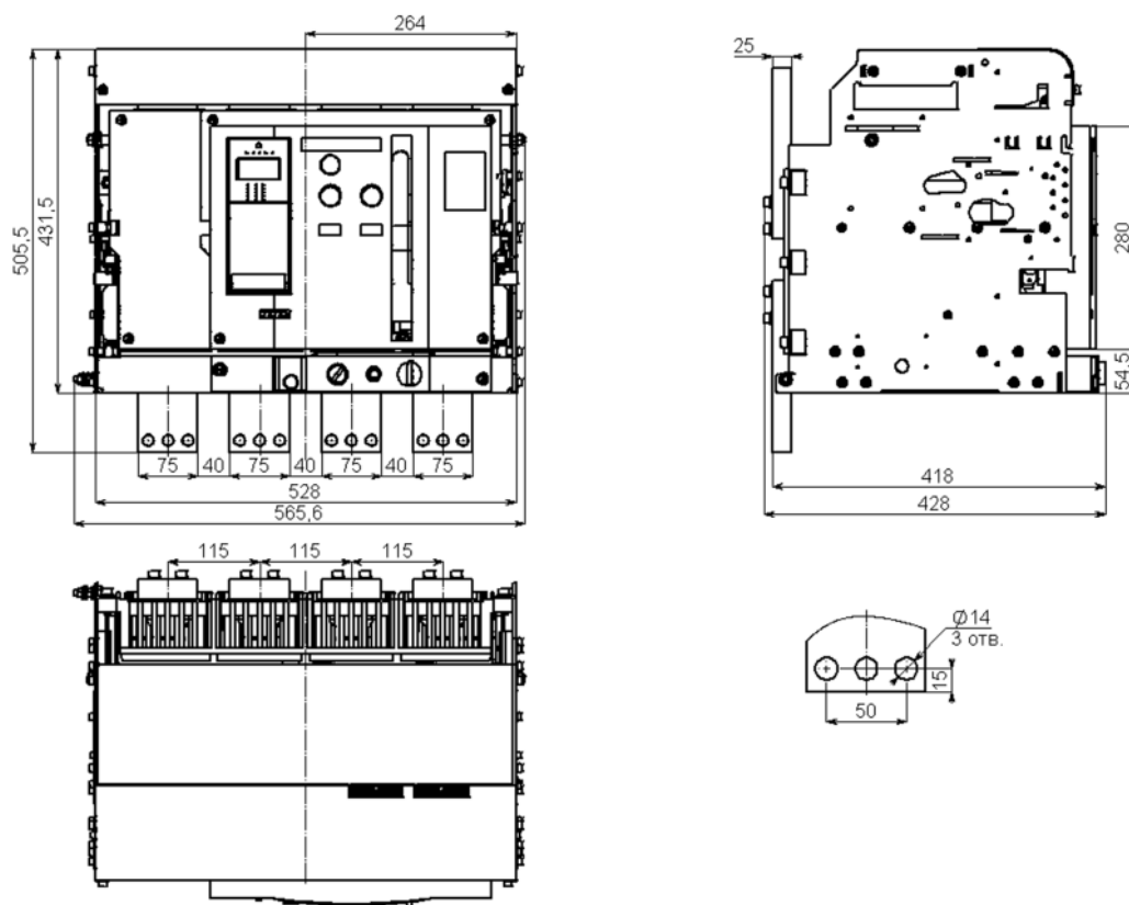
Рисунок А.20 – Автоматический выключатель YON AD-S4 выдвижного исполнения на номинальные токи 2500–3200 А переднего присоединения 4 полюса
