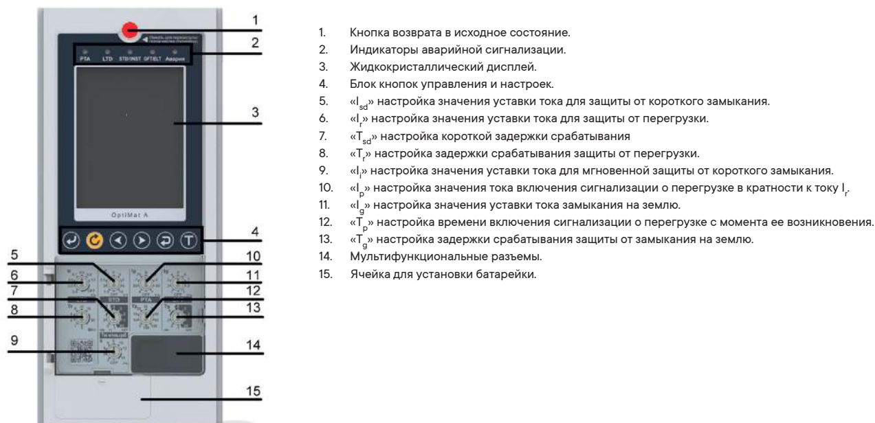
Рисунок 24 – Микропроцессорный расцепитель MR8.2
