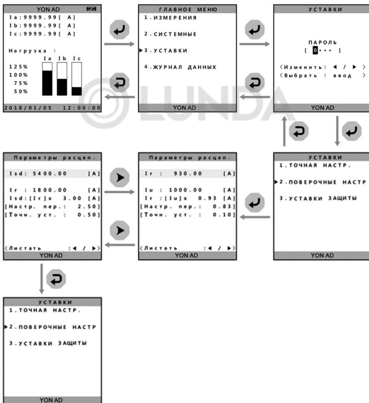
Рисунок 22 – «Поверочные настройки»
