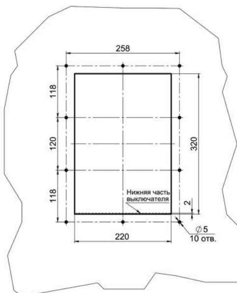
Рисунок А.8 – Вырез в дверце для автоматического выключателя YON AD630-1600-S1 выдвижного исполнения
