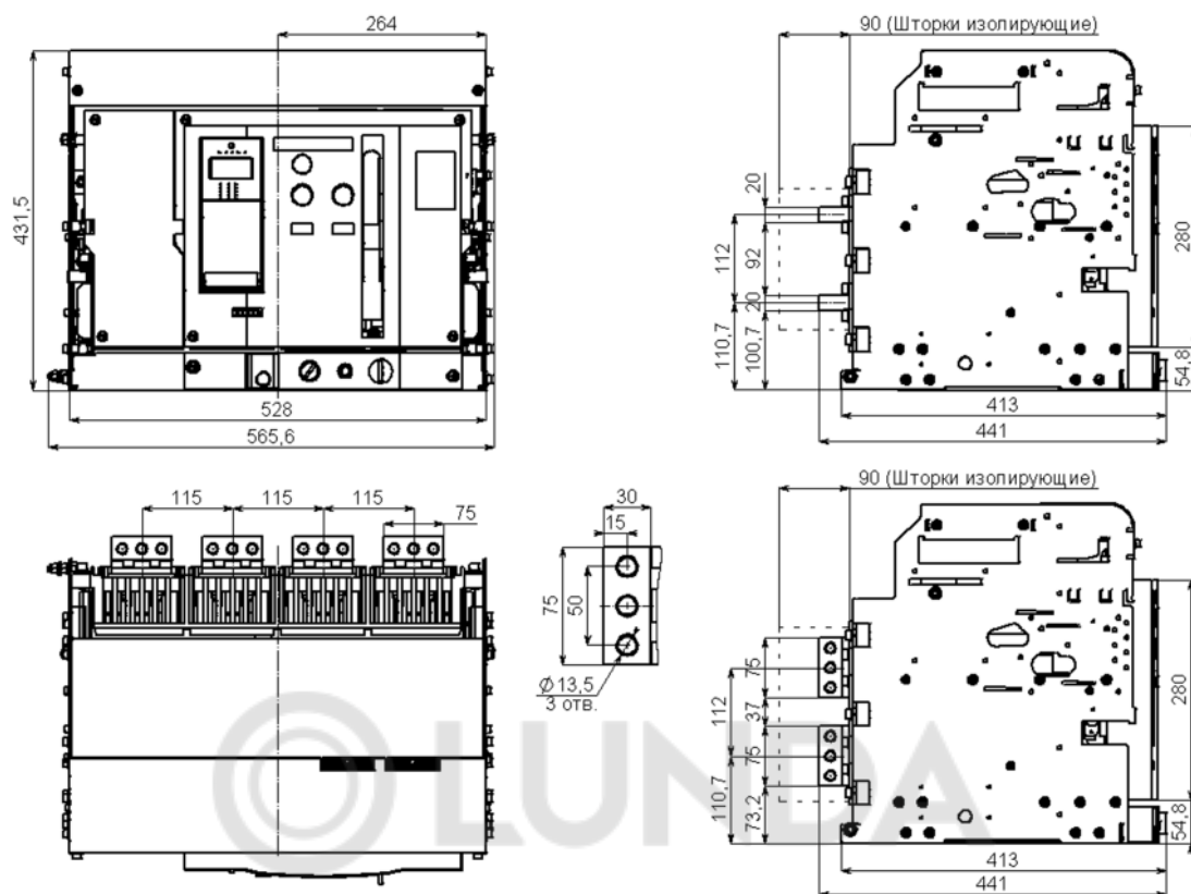
Рисунок А.19 – Автоматический выключатель YON AD-S4 выдвижного исполнения на номинальные токи 2500–3200 А заднего присоединения 4 полюса
