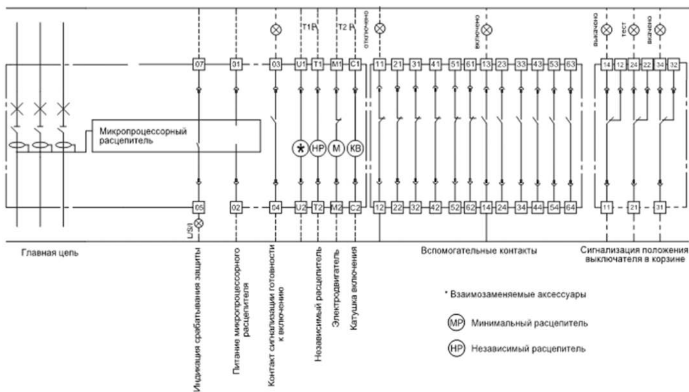
Рисунок В.2 – Принципиальная электрическая схема выключателя с микропроцессорным расцепителем типа MR7.0
