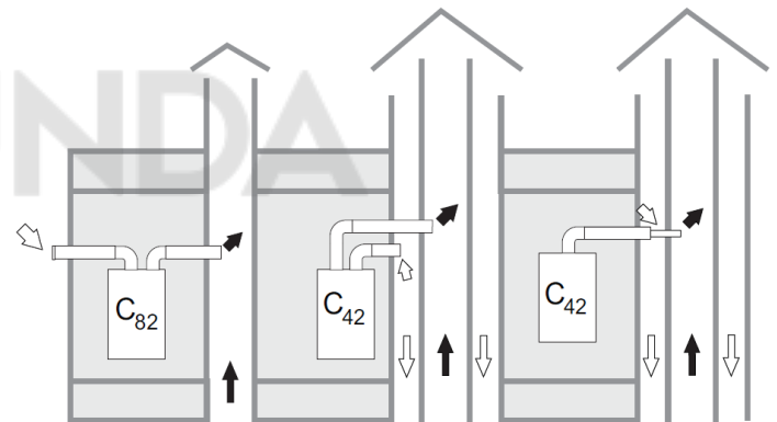
Рис. 6. Примеры систем дымоудаления собранных с помощью отдельных труб. Белой стрелкой обозначен приток воздуха, черной стрелкой поток продуктов сгорания.
