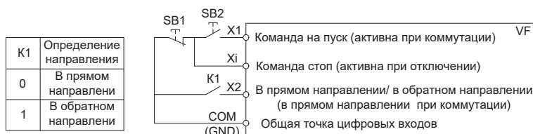
Рисунок 10.9-7. Трехпроводная схема управления 1
