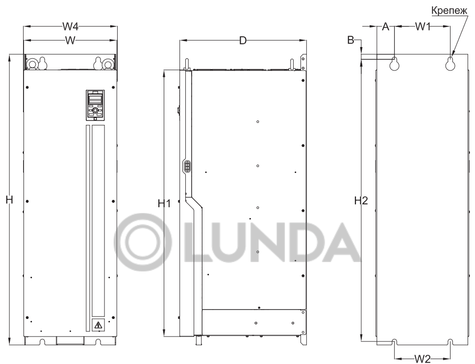
Рисунок 3.6-11. Чертеж преобразователя частоты типоразмер В11
