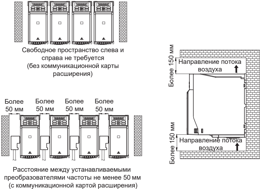
Рисунок 3.5-1. Положение преобразователя частоты и необходимое пространство
