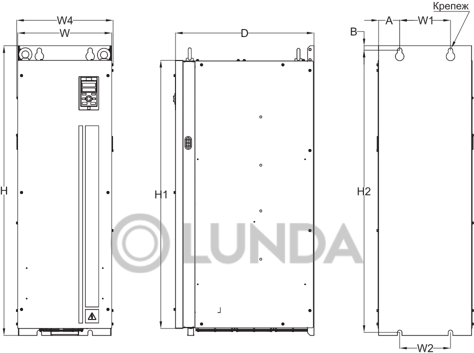
Рисунок 3.6-10. Чертеж преобразователя частоты типоразмер B10
