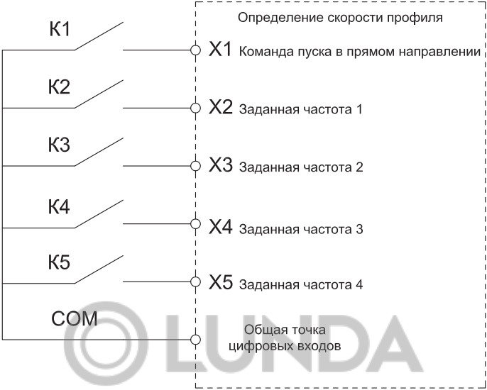
Рисунок 10.18-1. Схема подключения клемм
