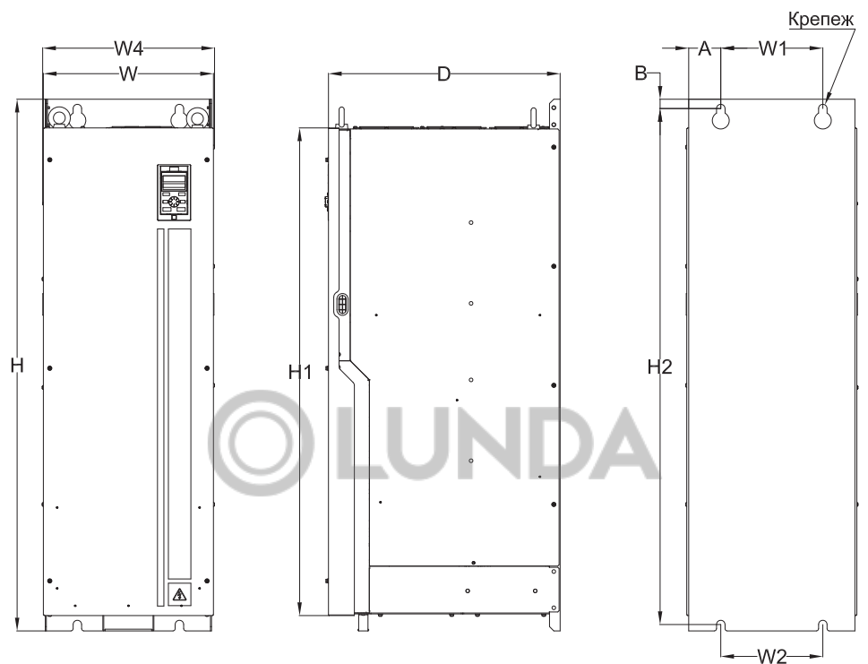
Рисунок 3.6-11. Чертеж преобразователя частоты типоразмер B11
