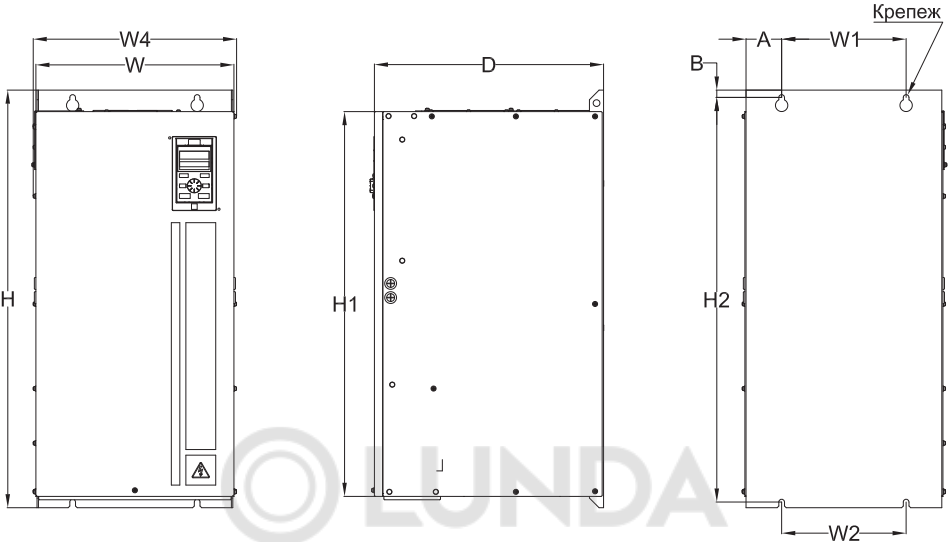
Рисунок 3.6-8. Чертеж преобразователя частоты типоразмер B8
