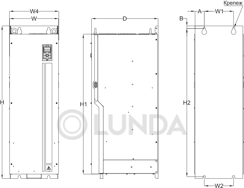
Рисунок 3.6-11. Чертеж преобразователя частоты типоразмер B11
