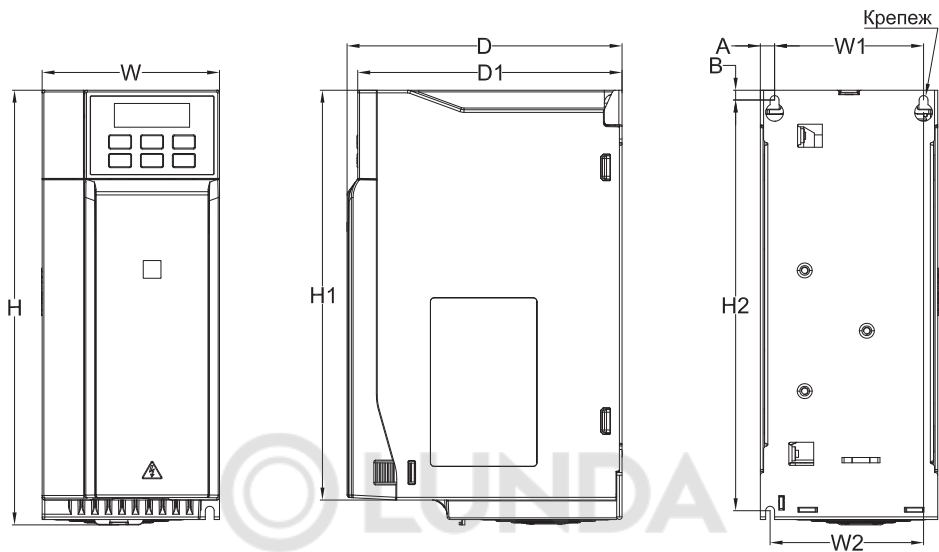
Рисунок 3.6-2. Чертеж преобразователя частоты типоразмер B2
