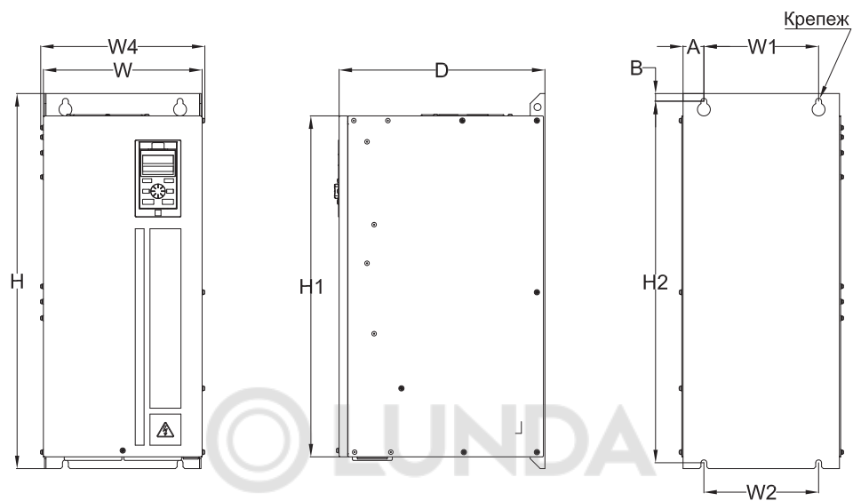
Рисунок 3.6-7. Чертеж преобразователя частоты типоразмер В7
