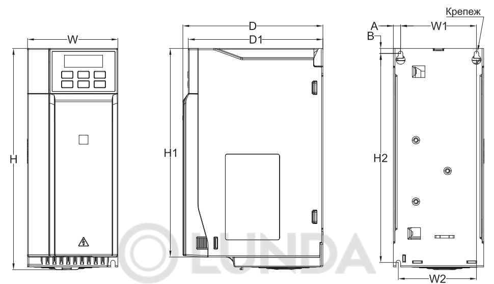
Рисунок 3.6-2. Чертеж преобразователя частоты типоразмер В2
