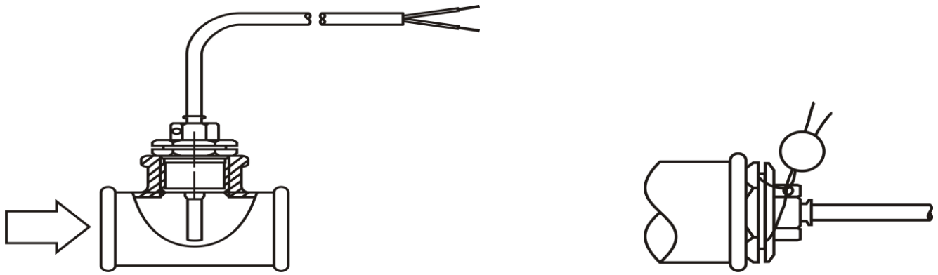
Рис. 4. Монтаж термомпреобразователя сопротивления в штуцере при помощи ниппеля и пломбирование.
