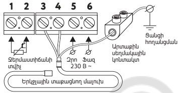
Նկ 2. Էլեկտրական ցանցին ներքևակի միացման սխեմա
