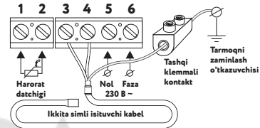
2-rasm. To'shakni elektr tarmog'iga ulash sxemasi
