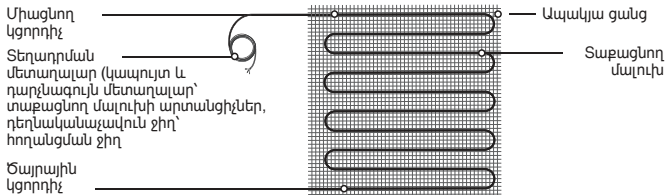
Նկ 1. Ներքևակի կառուցվածքը
