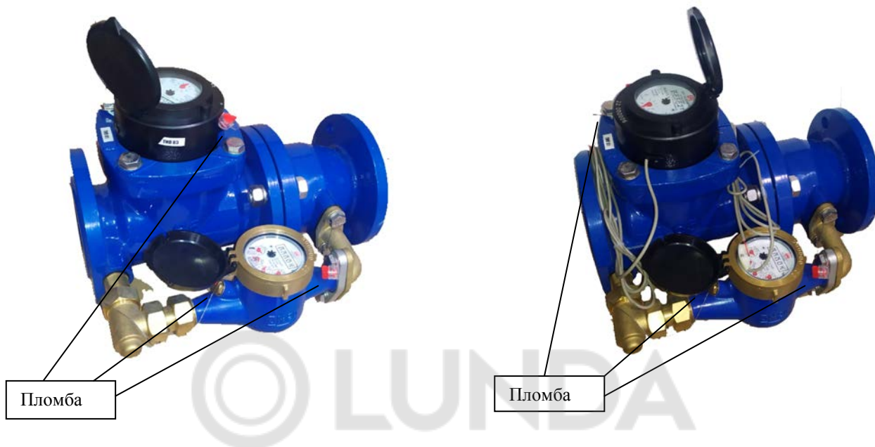
Рисунок А1. Внешний вид и опломбировка счётчиков КВСХ-01, КВСХд-01
