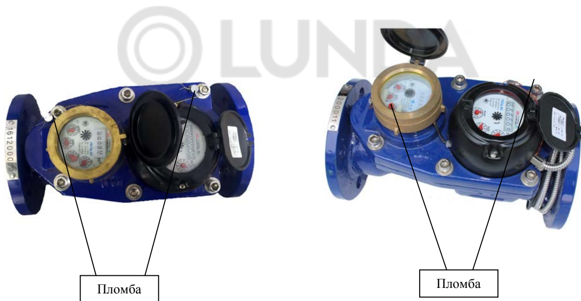
Рисунок А4. Внешний вид и опломбировка счётчиков КВСХ-04, КВСХд-04.
