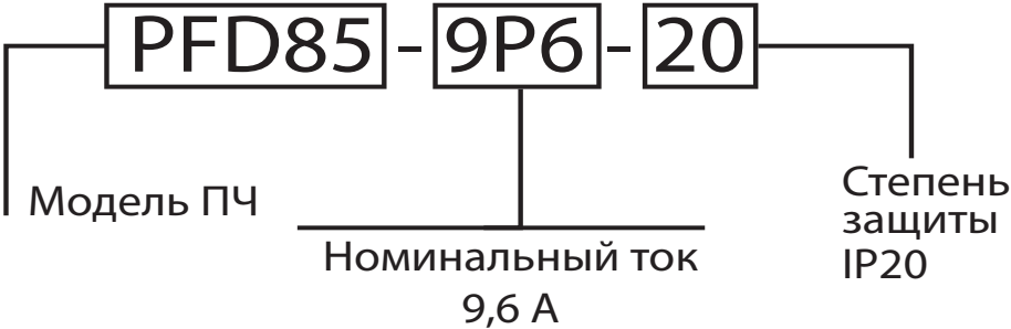
Рис. 2.1 Маркировка ПЧ
