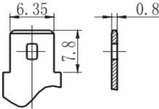
Рисунок А2. Внешний вид и габаритные размеры выводов подключения внутренних АБ
