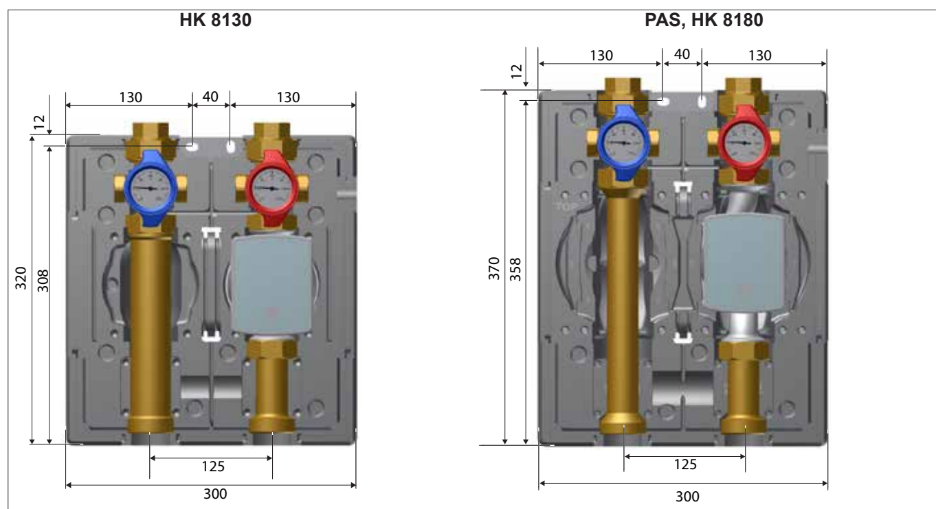
Рис. 2: Размеры (мм)
