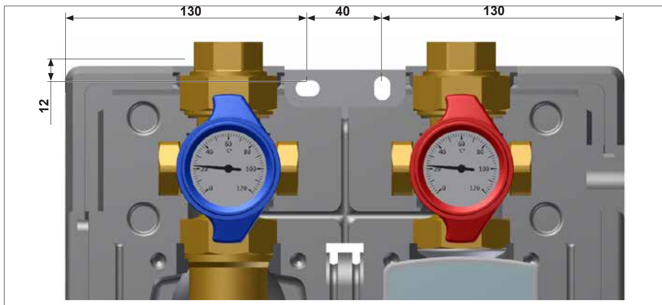
Рис. 4: Маркировка [мм]
