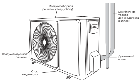
Рис. 2. Наружный блок*.
