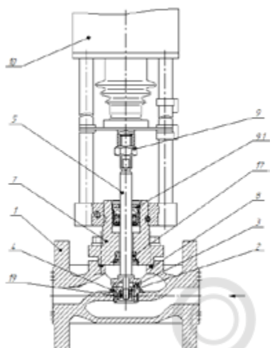
Рисунок 2. Неразгруженный по давлению клапан DN 15 – 40. Исполнение А.
