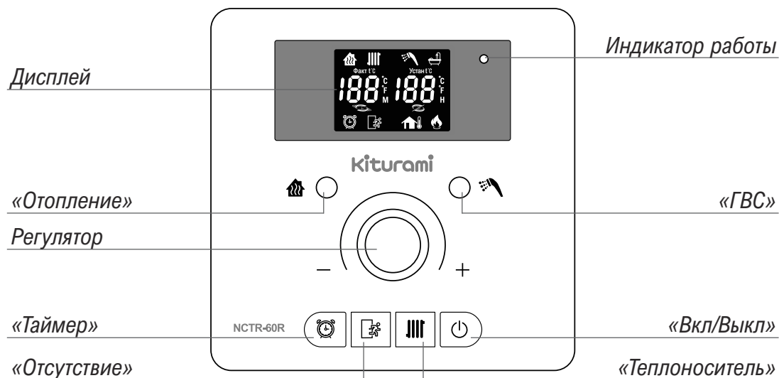
Рисунок 8. Дисплей и кнопки управления NCTR-60R.
