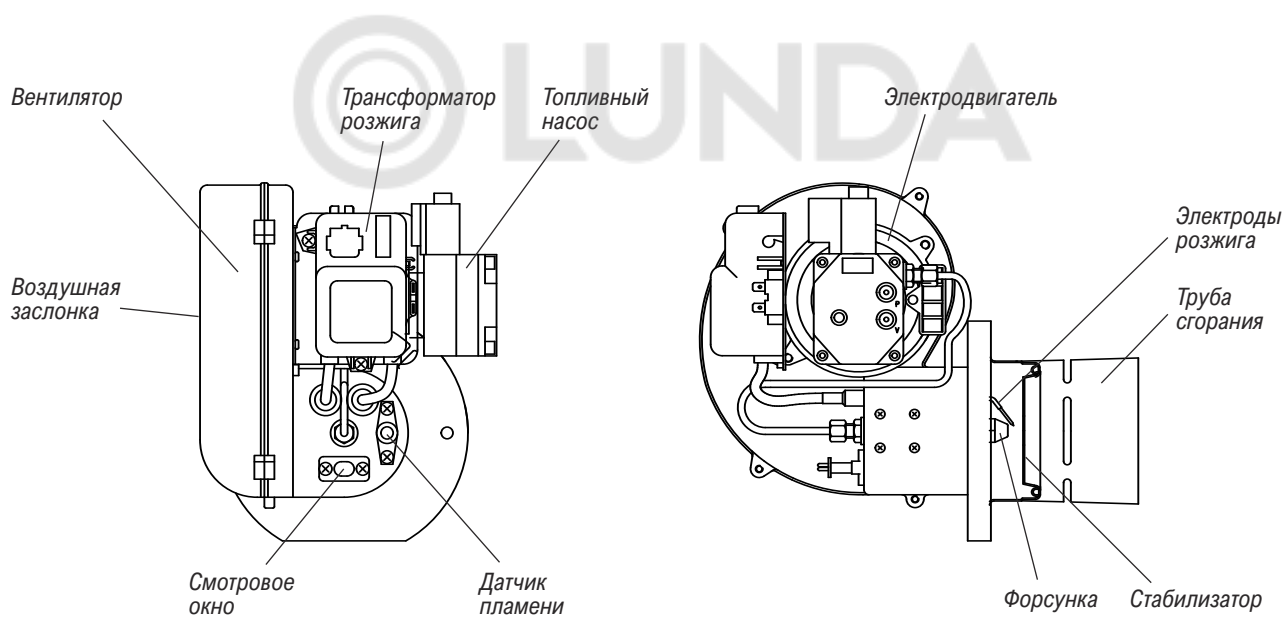
Рисунок 4. Основные горелки Turbo 15/20.
