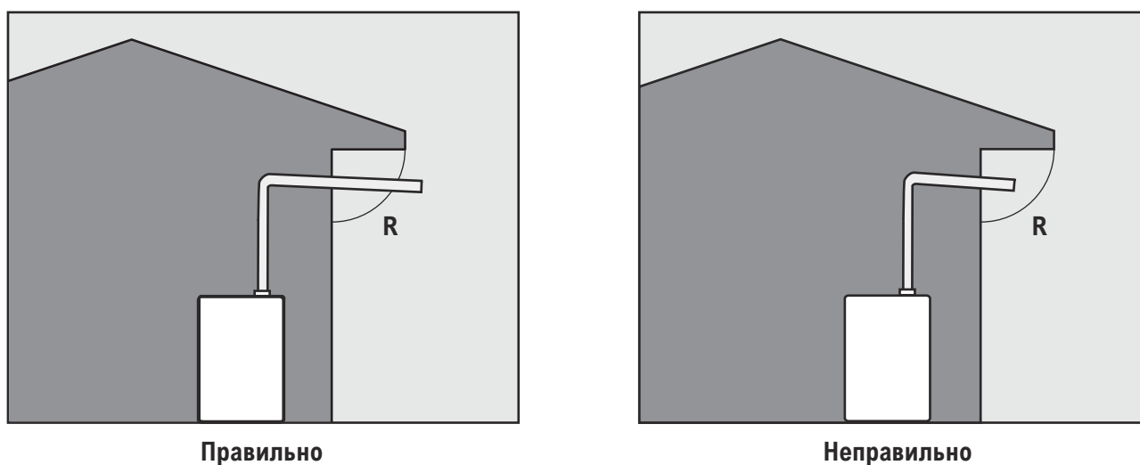
Рисунок 12. Зона повышенного давления воздуха.
